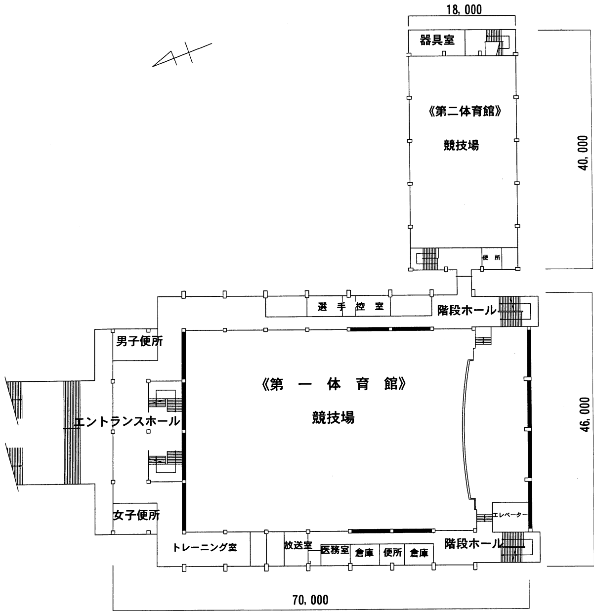
2階平面図
