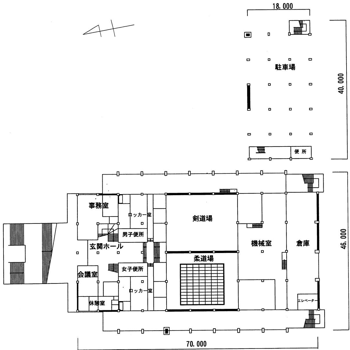
1 階平面図
