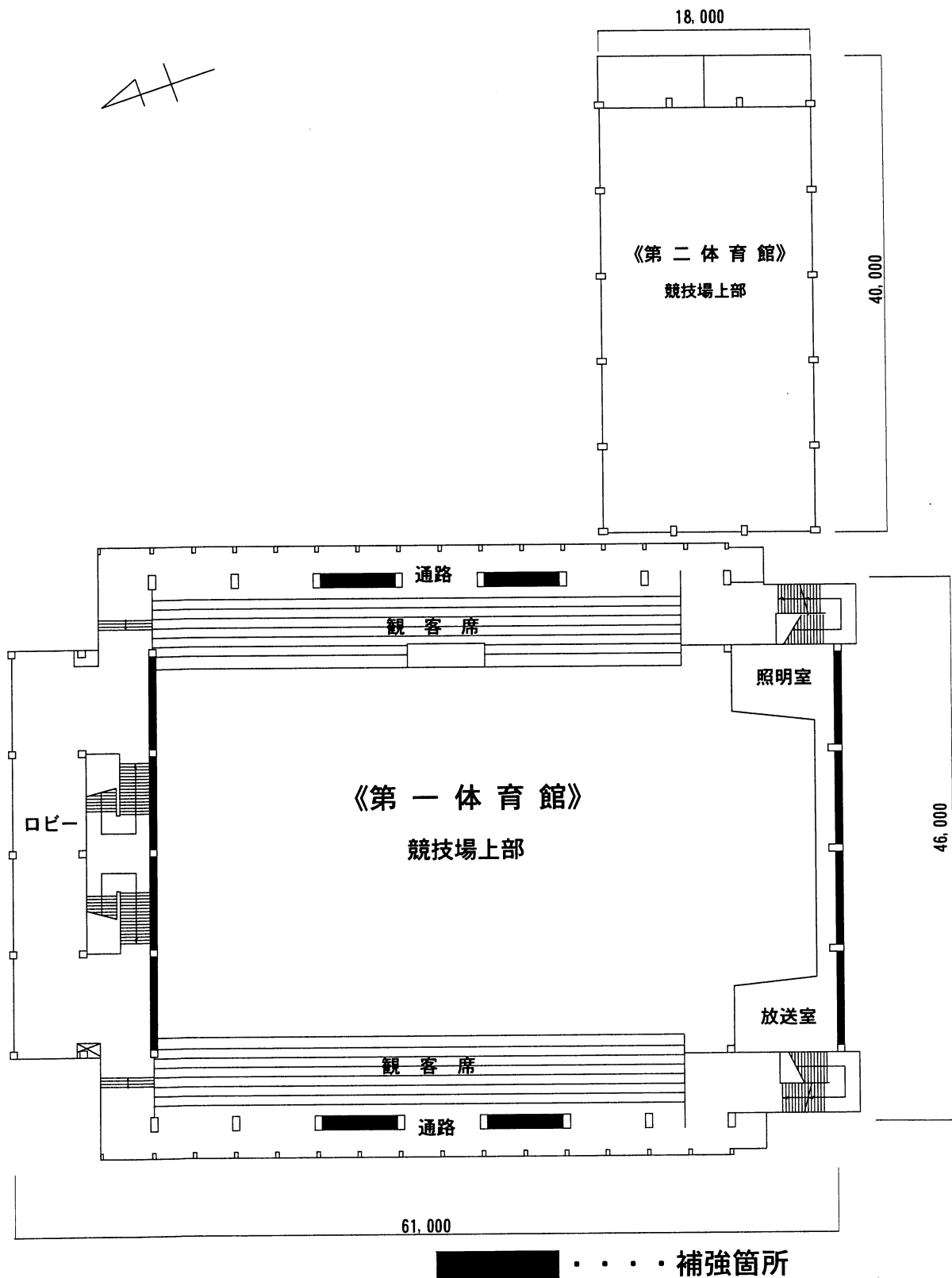
3階平面図
