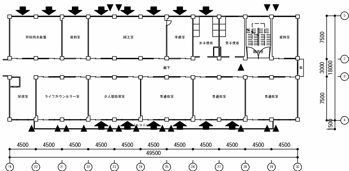
2 階平面図
