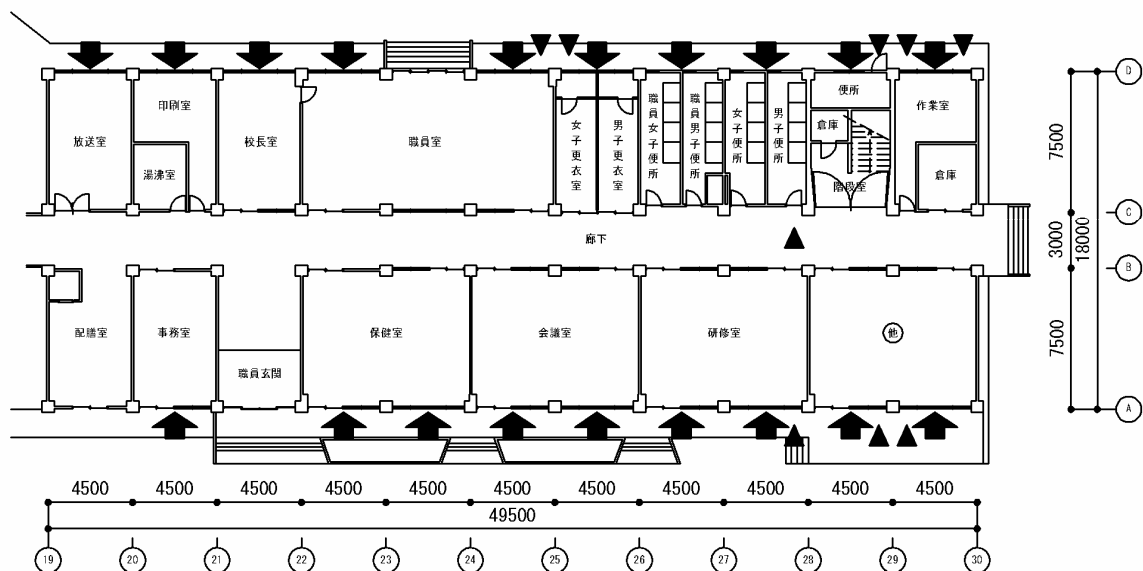
1 階平面図
