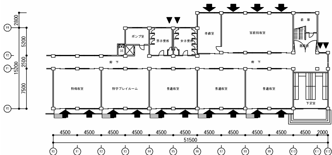
1 階平面図
