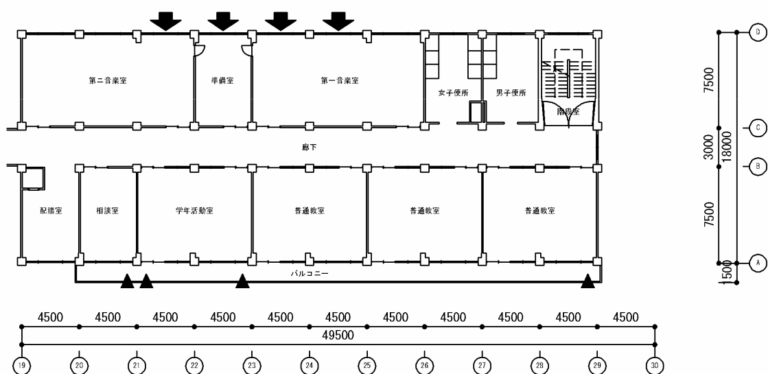
4 階平面図
