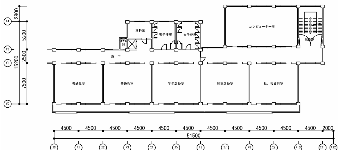
4 階平面図
