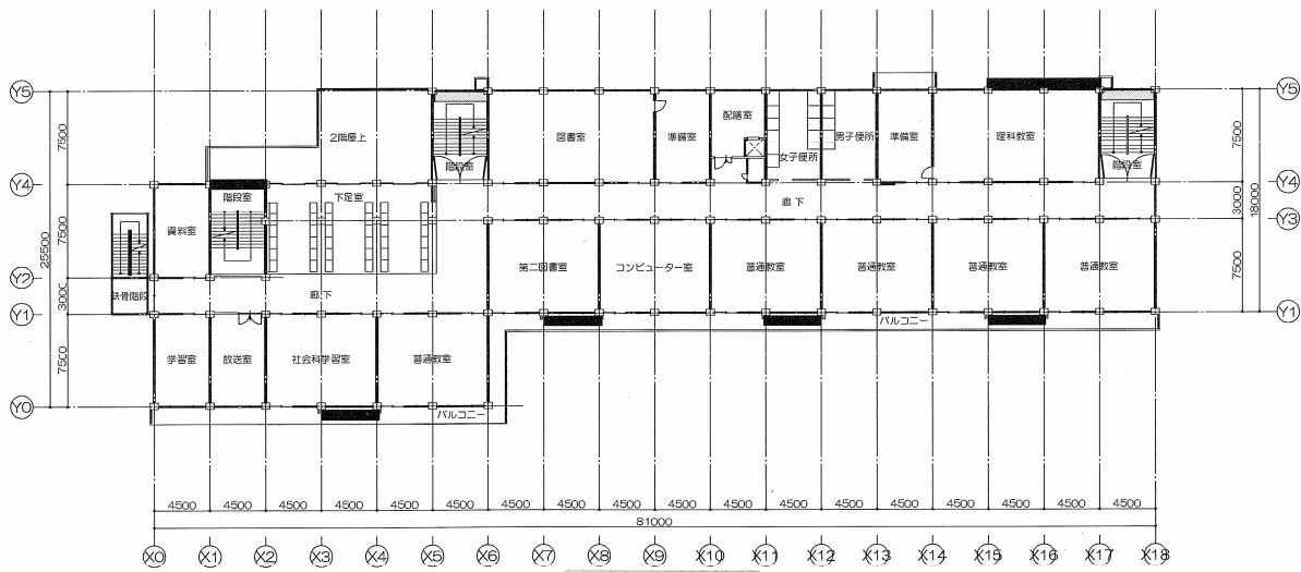
2階平面図
