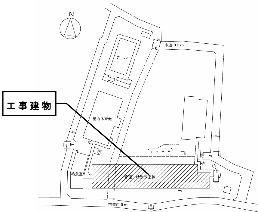
配置図
