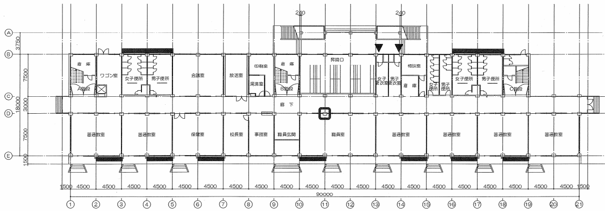
1階平面図
