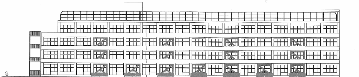
南立面図
