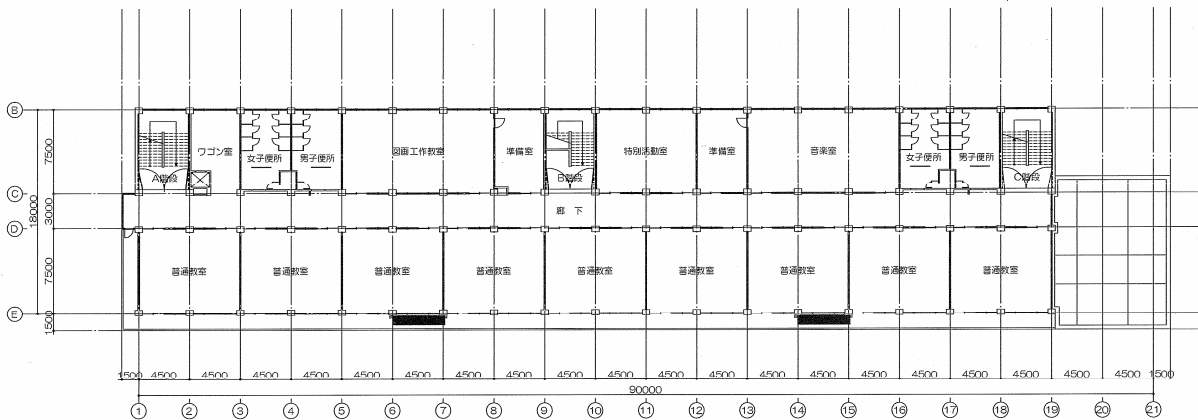
4階平面図
