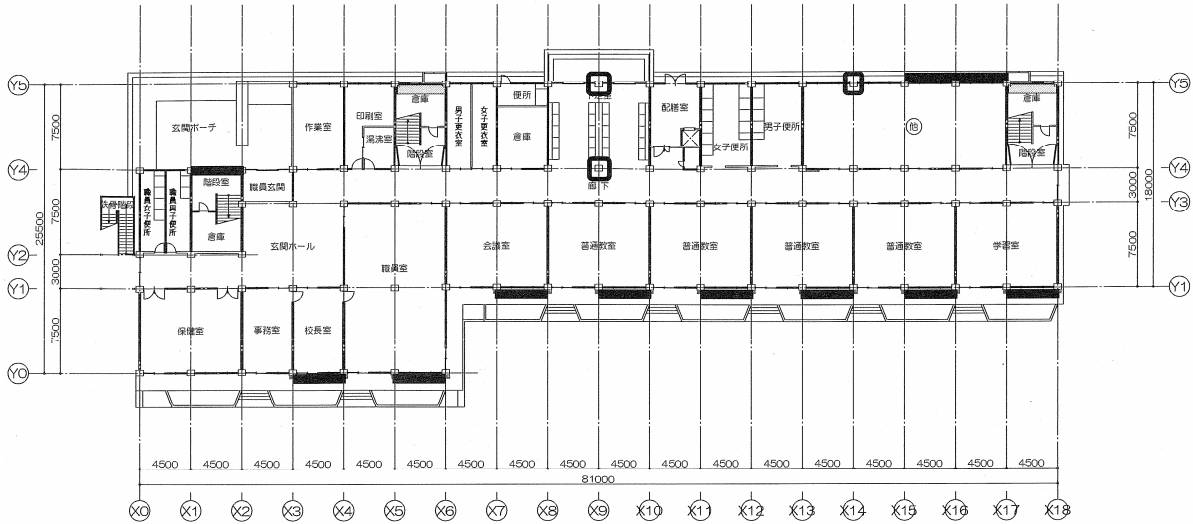
1階平面図
