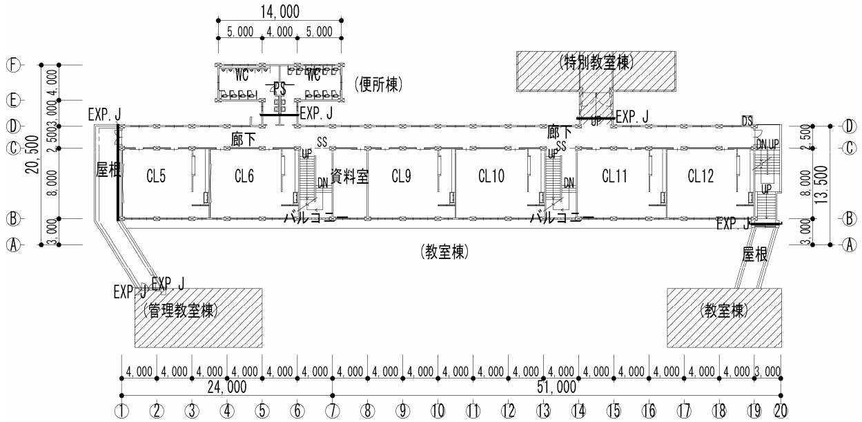
3階平面図
