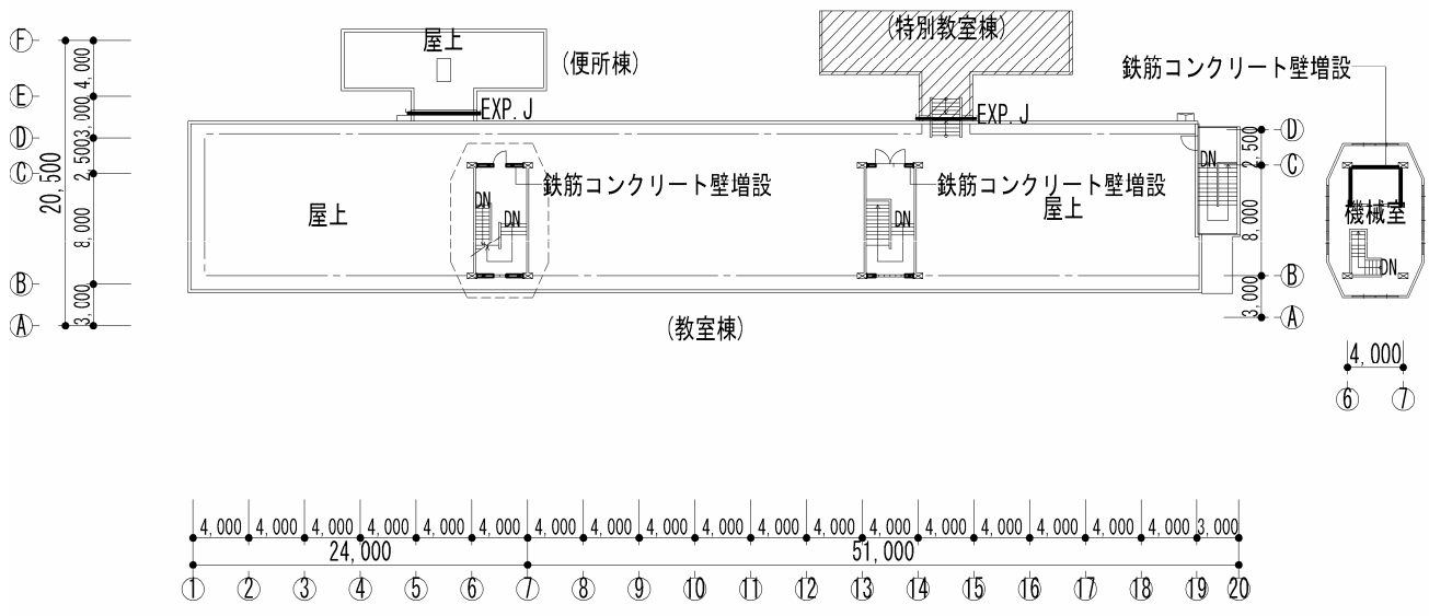
R階平面図
