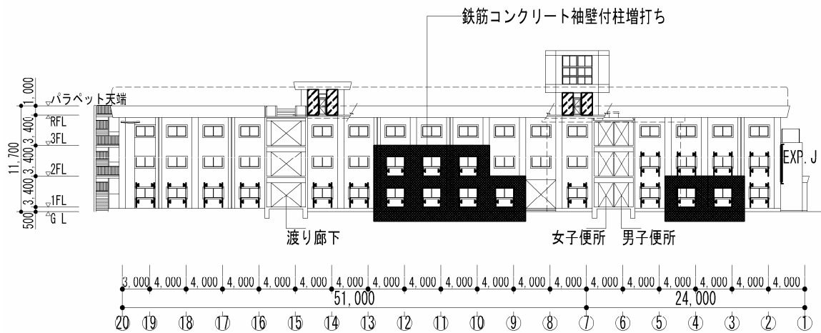
北側立面図
