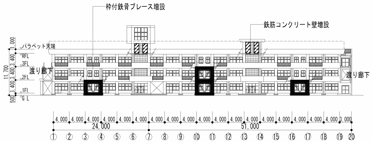
南側立面図
