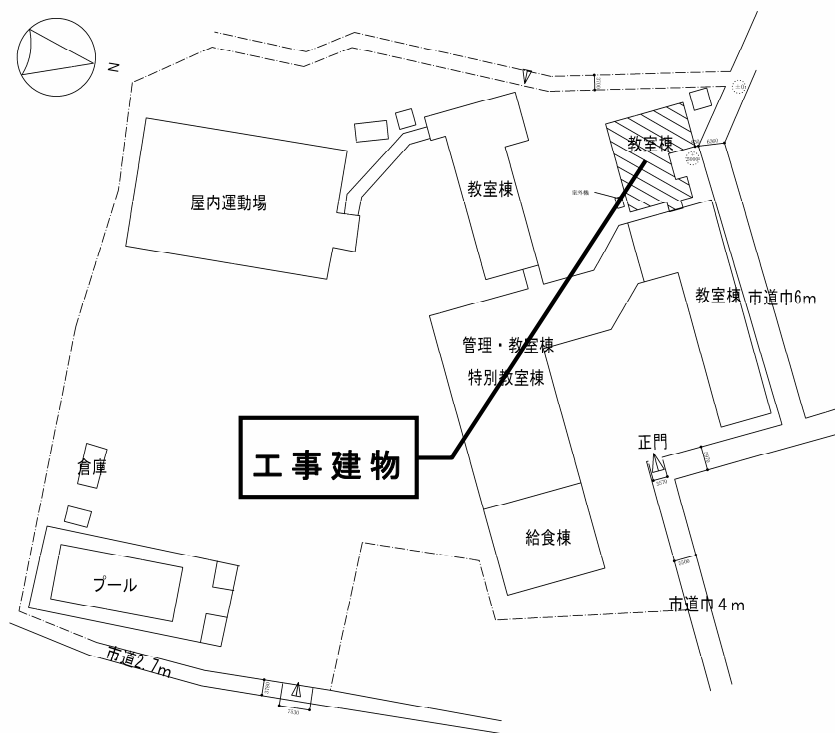
配置図
