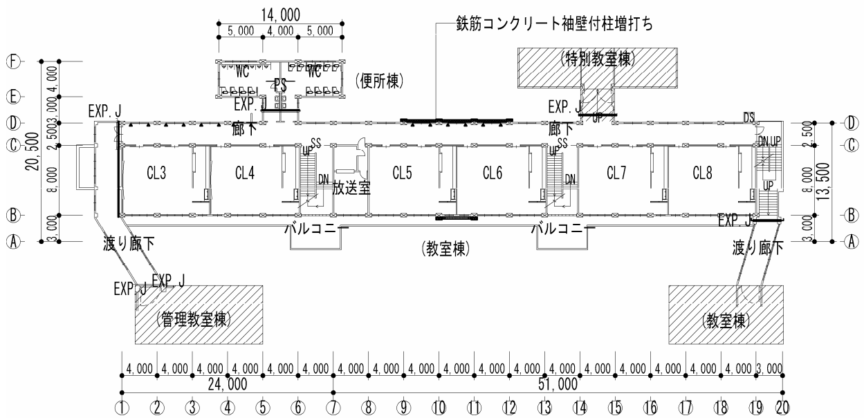
2階平面図
