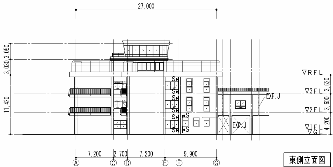
市川市立八幡小学校 耐震補強立面図
