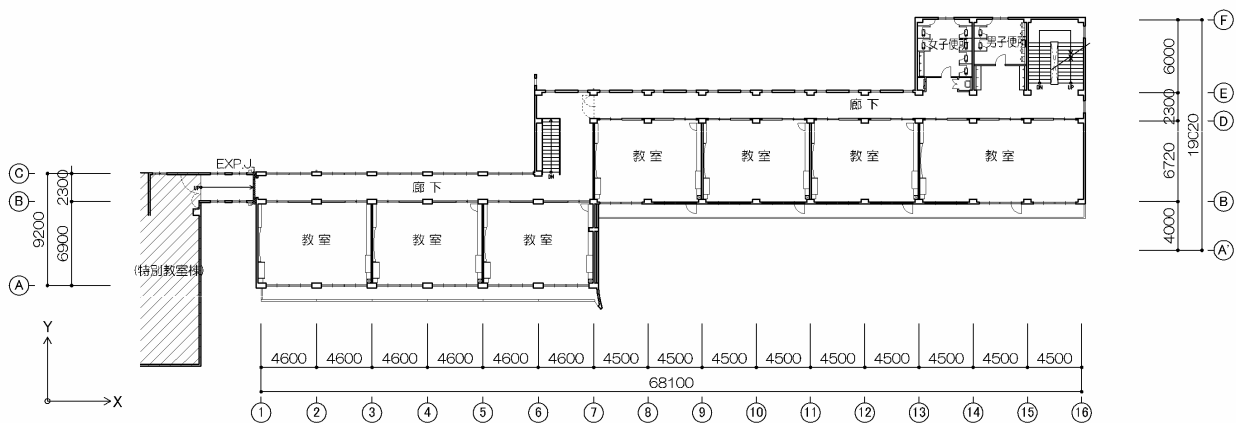
3 階平面図
