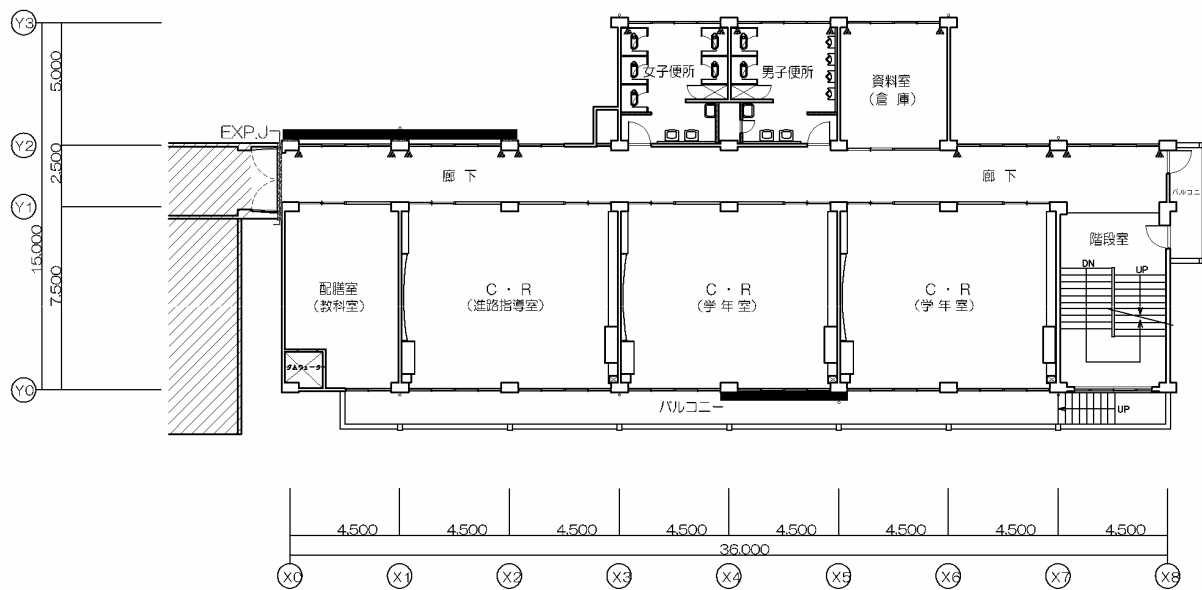
3階平面図
