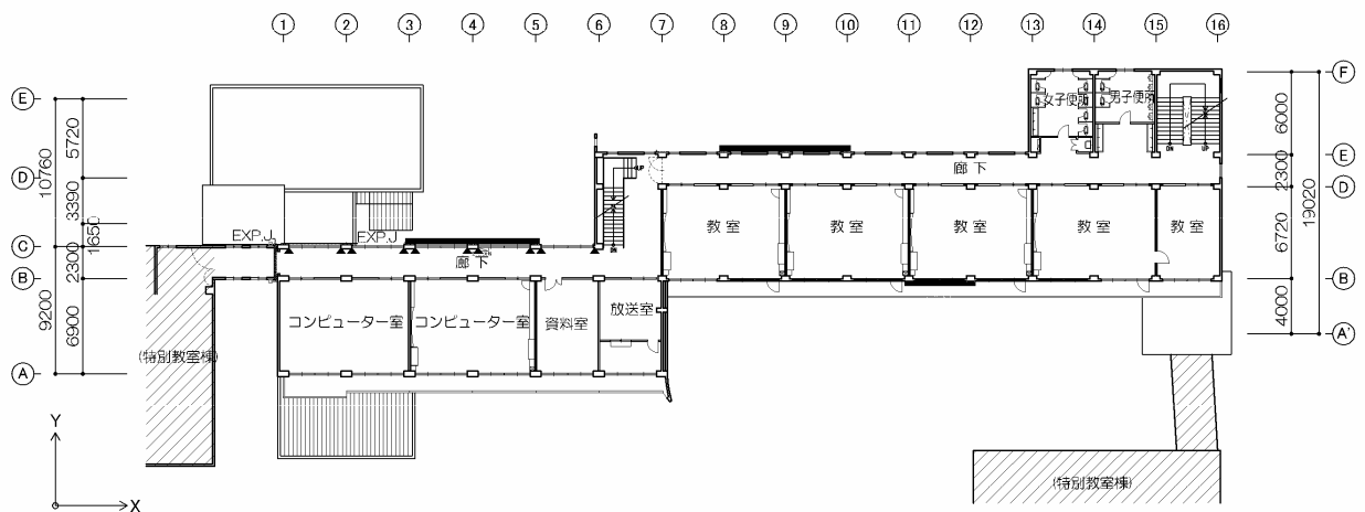
2階平面図
