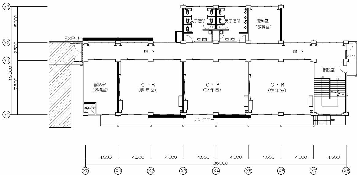
2階平面図
