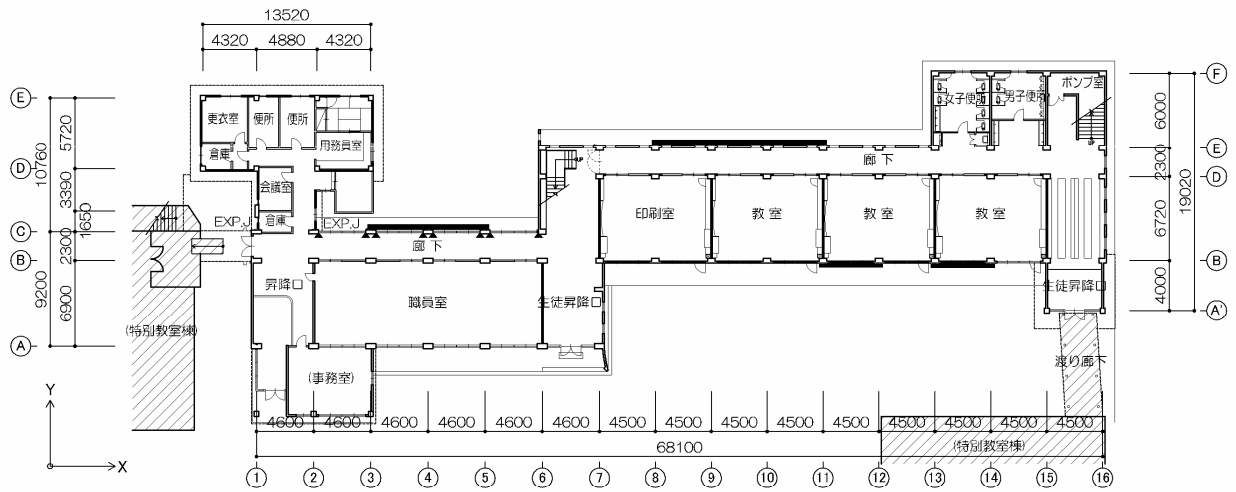
1階平面図
