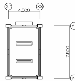
塔屋平面図
