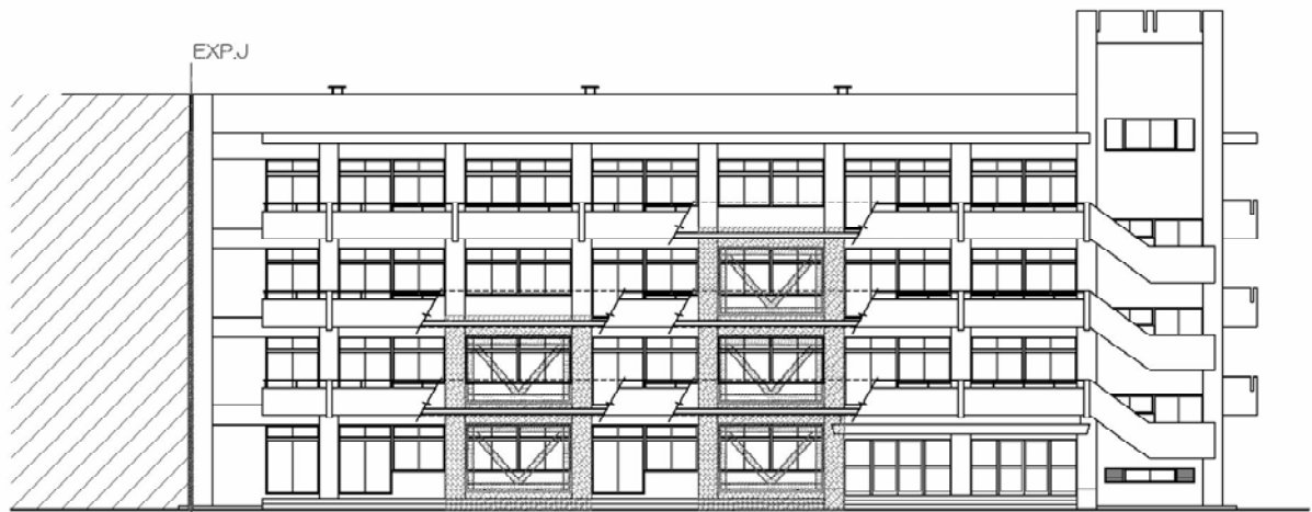
南側立面図
