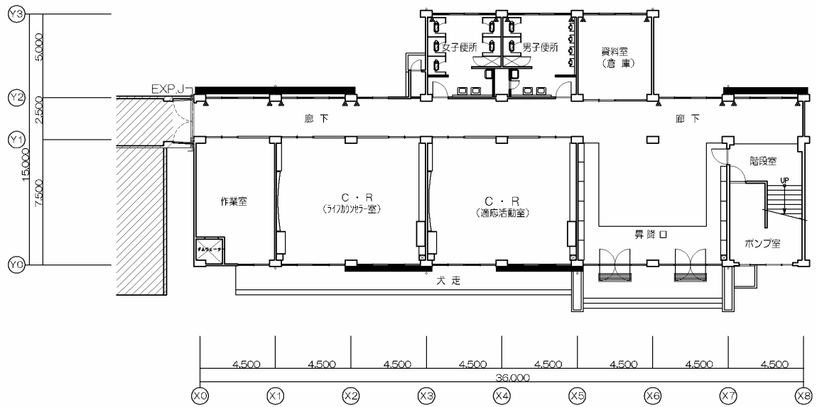
1階平面図
