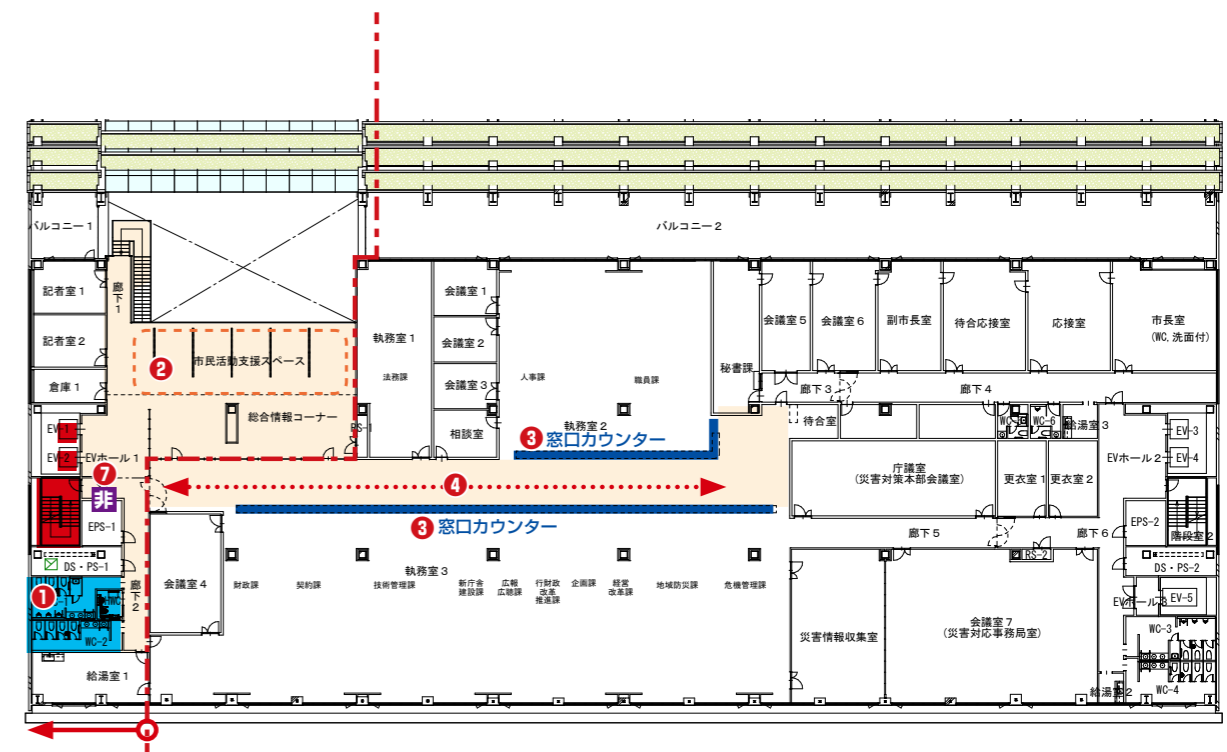
4階平面図
