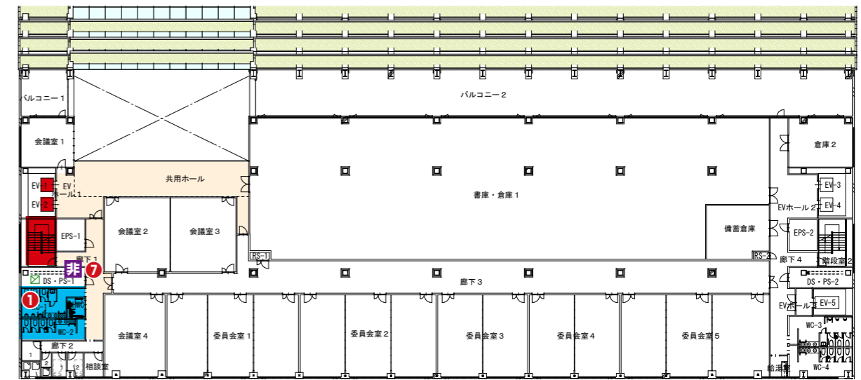
5階平面図
