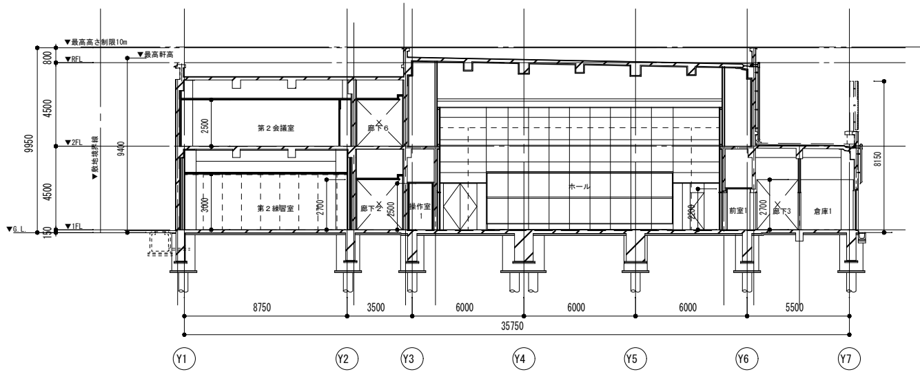
B-B断面図
