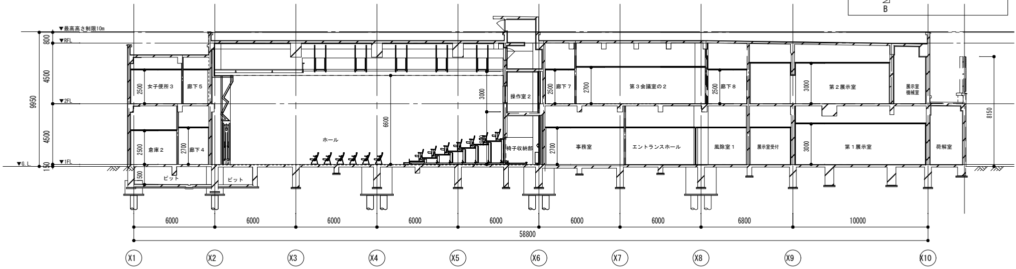
A-A断面図
