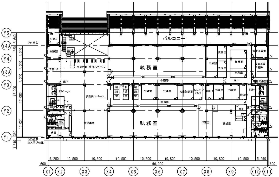
3階平面図
