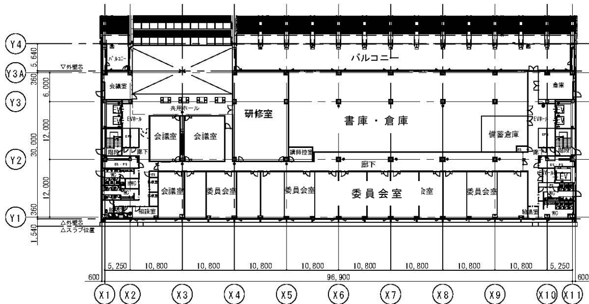
5階平面図
