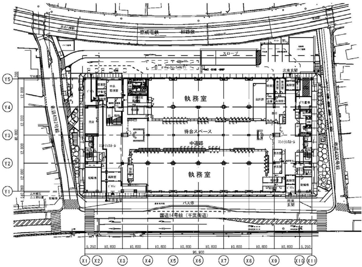
1階平面図
