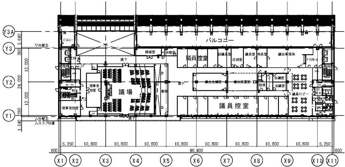
6 階平面図
