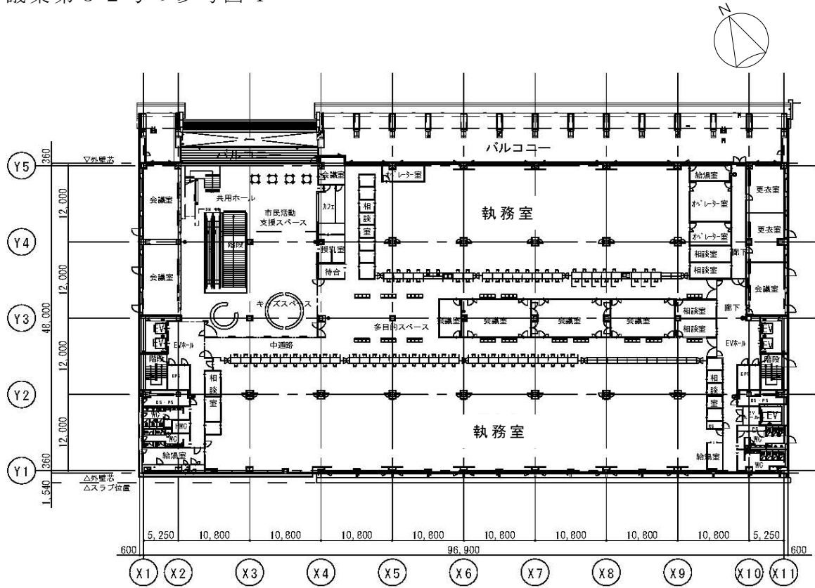
2階平面図
