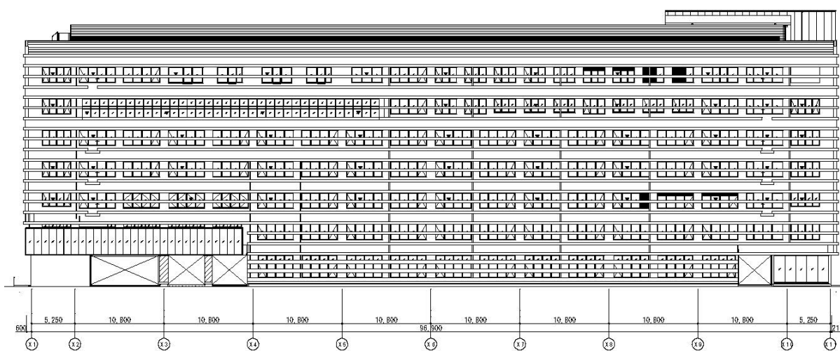
南立面図
