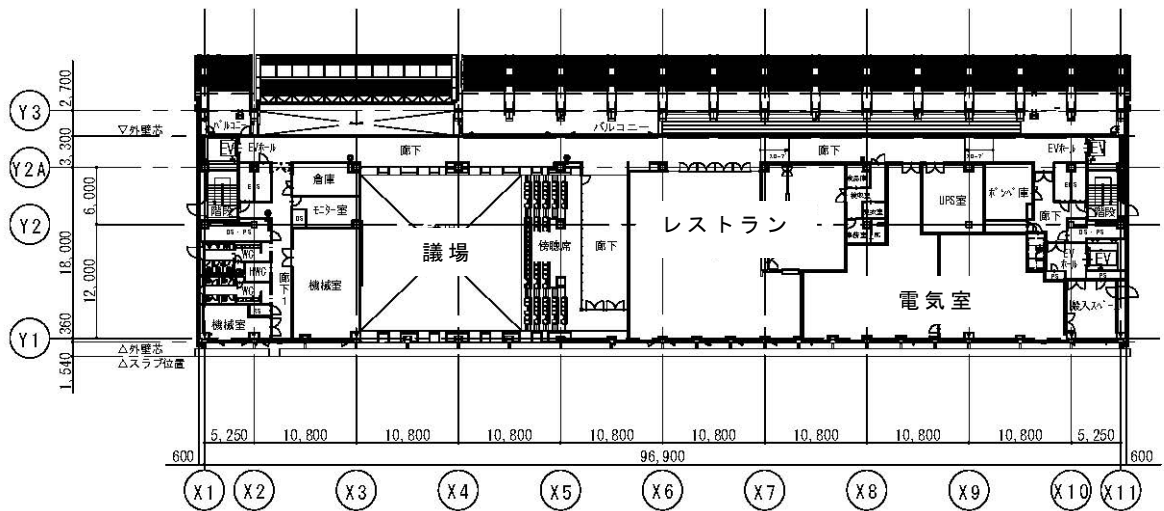
7 階平面図
