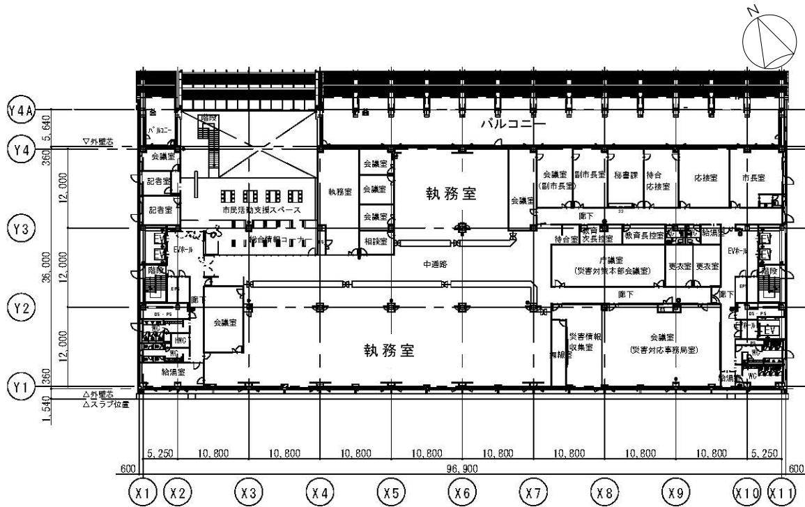
4階平面図
