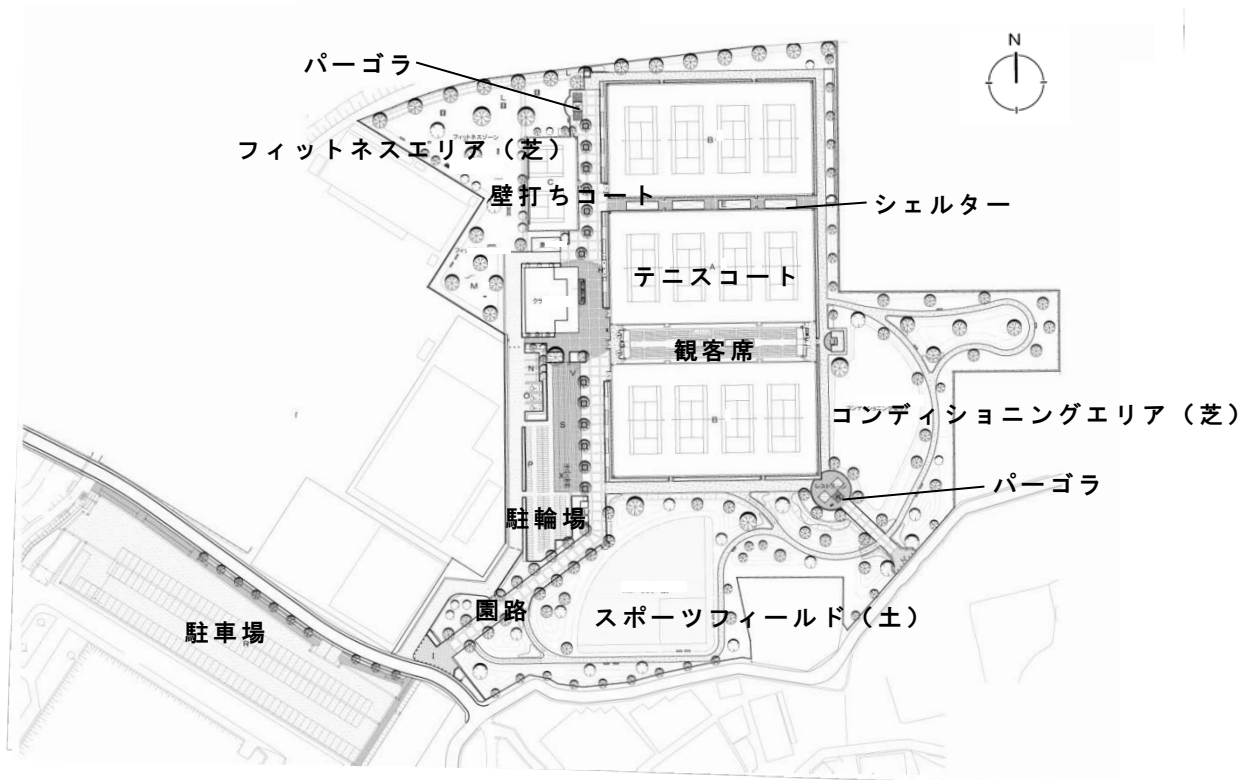
対象施設 配置図
