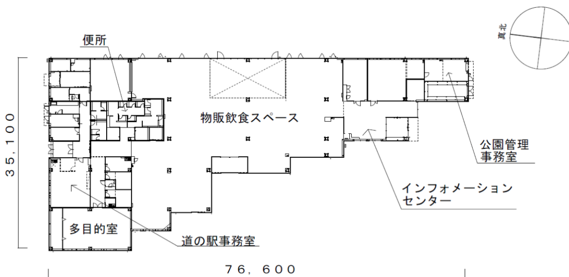
1 階平面図
