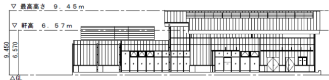
南立面図
