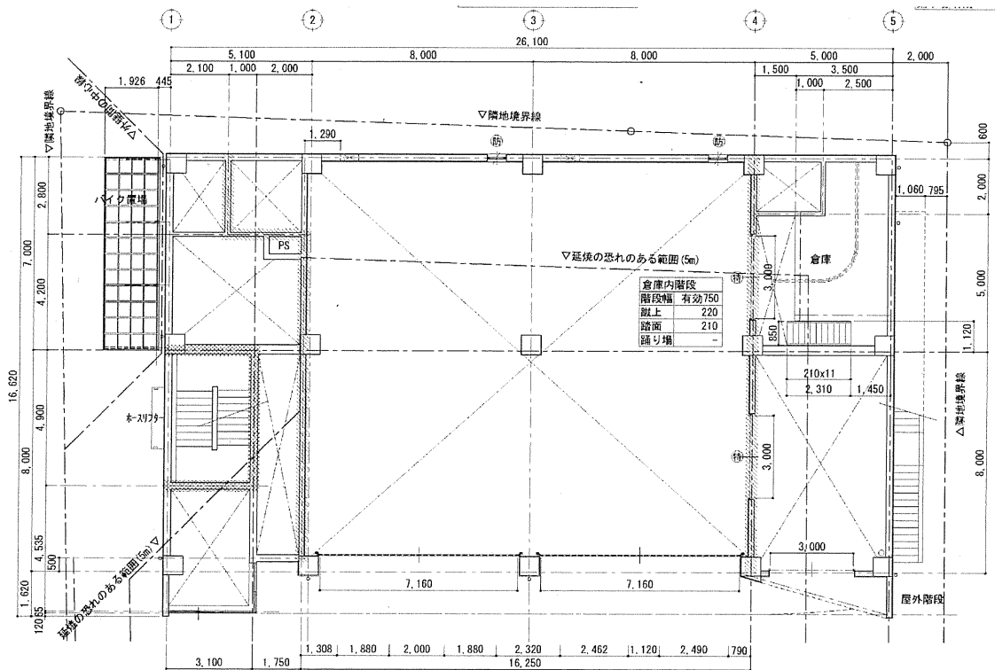
中2階平面図
