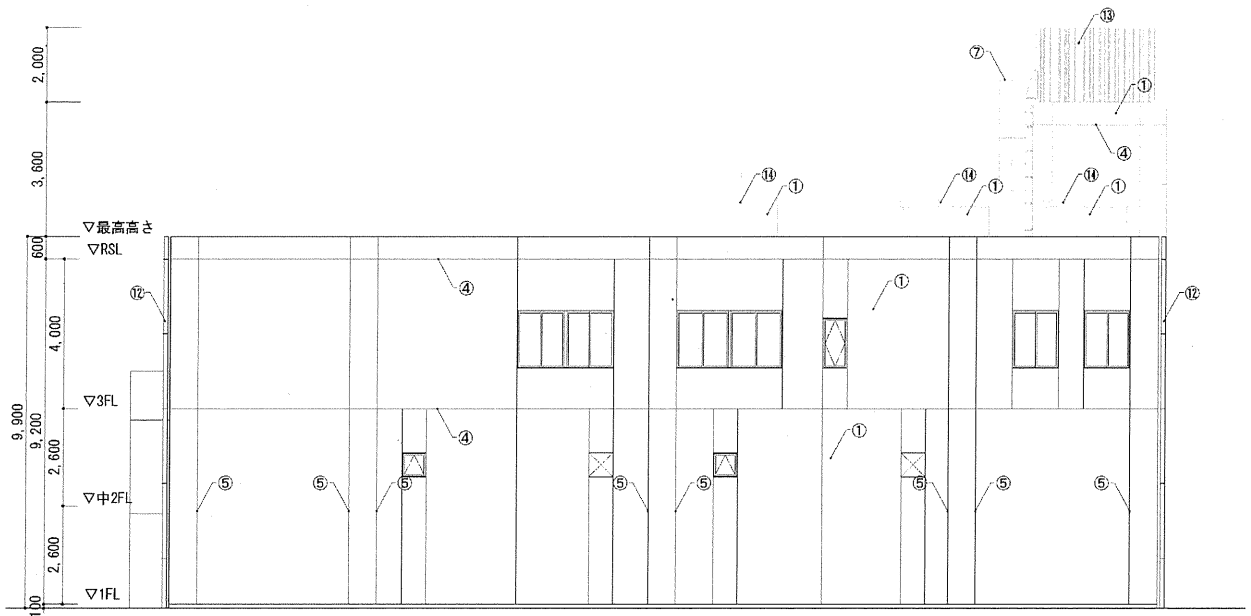
北側立面図
