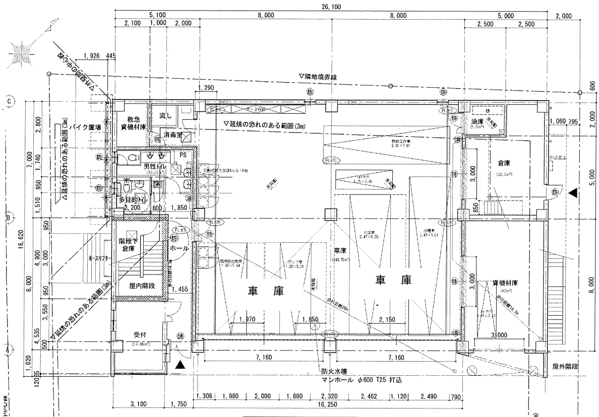
1階平面図
