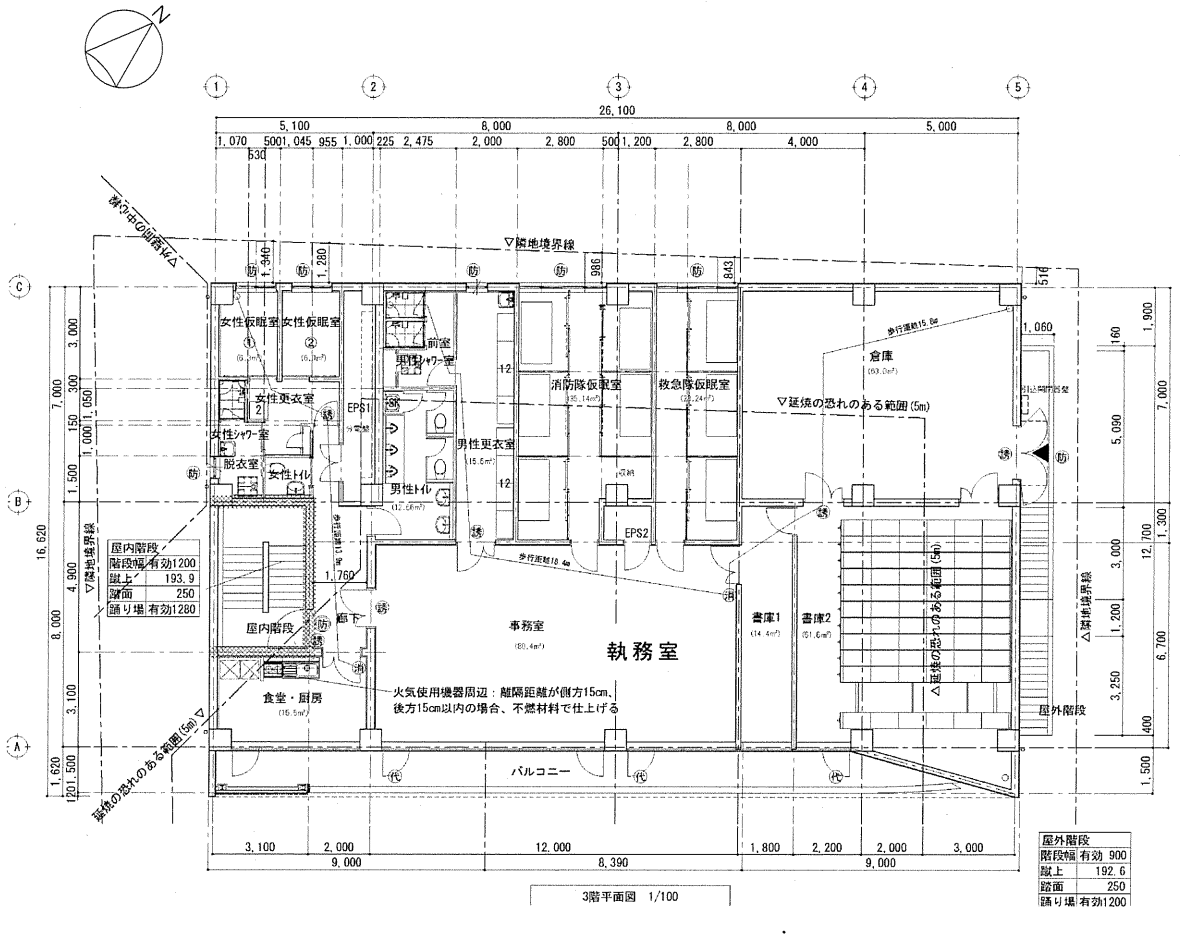
3階平面図
