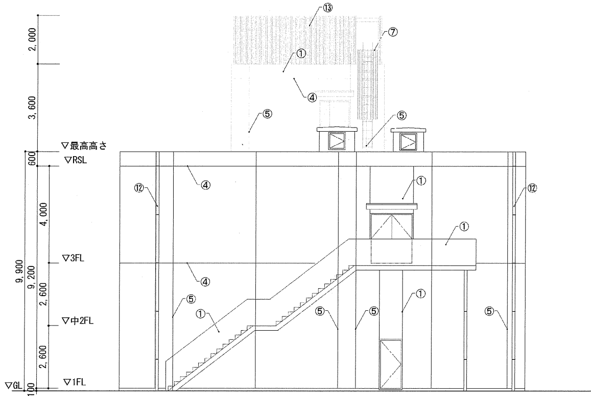
東側立面図
