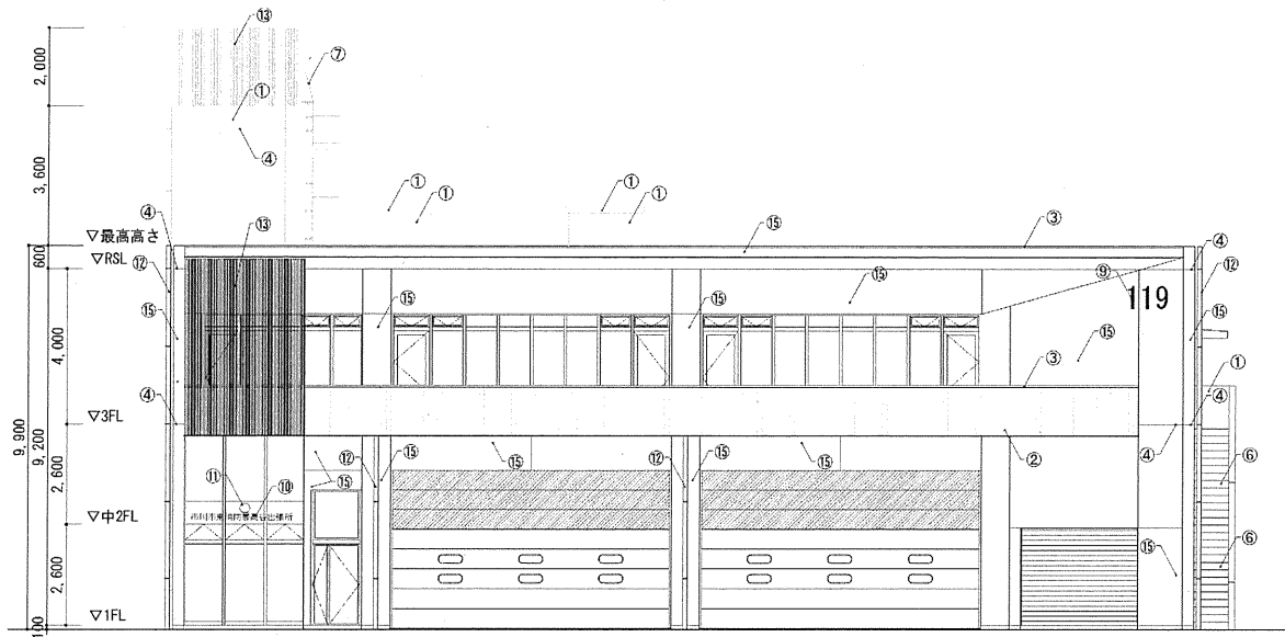
南側立面図
