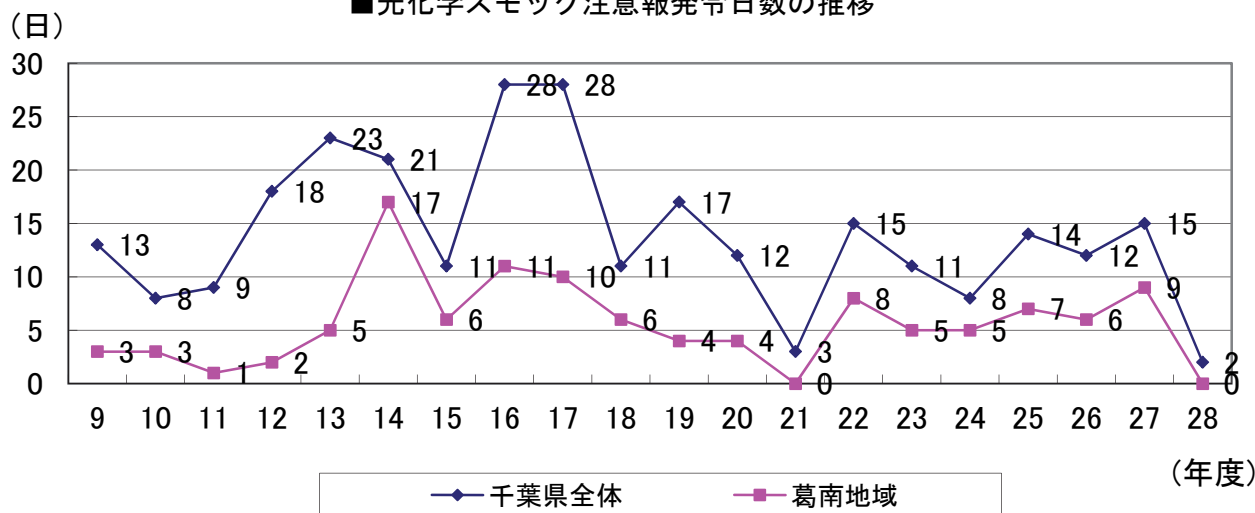
■光化学スモッグ注意報発令日数の推移
