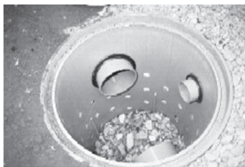
雨水浸透施設（浸透柵）
