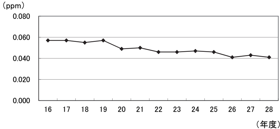
■二酸化窒素の日平均値の98%値の推移(市川市市川局)
