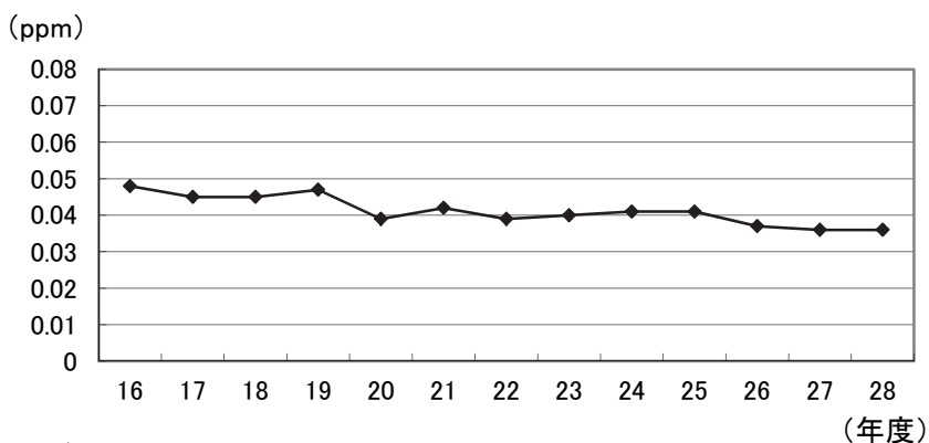
■ 二酸化窒素の日平均値の98%値の推移(市川本八幡局)
