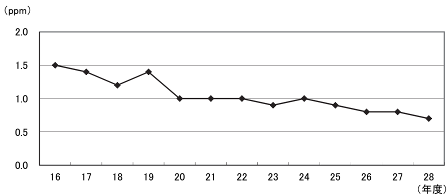
■一酸化炭素の日平均値の2%除外値の推移(市川市市川局)
