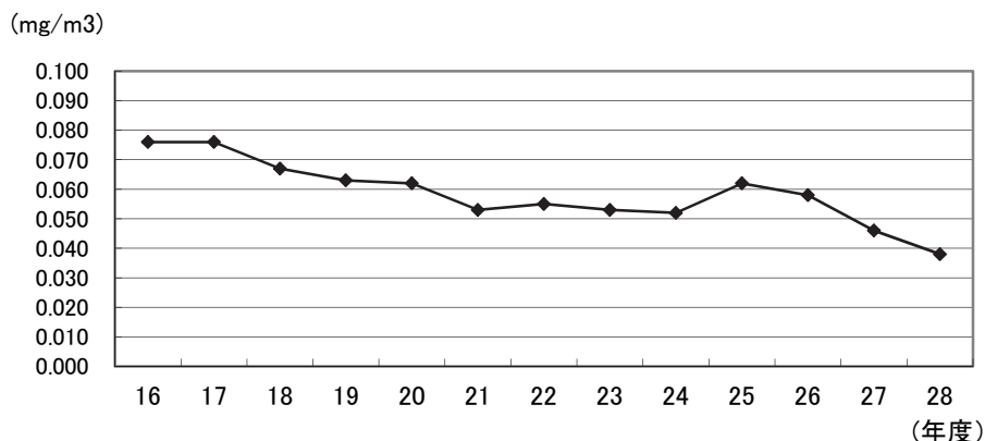
■浮遊粒子状物質の日平均値の2%除外値の推移(市川本八幡局)
