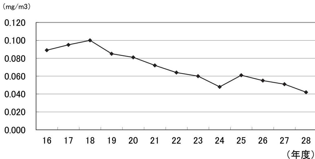
■浮遊粒子状物質の日平均値の2%除外値の推移(市川市市川局)
