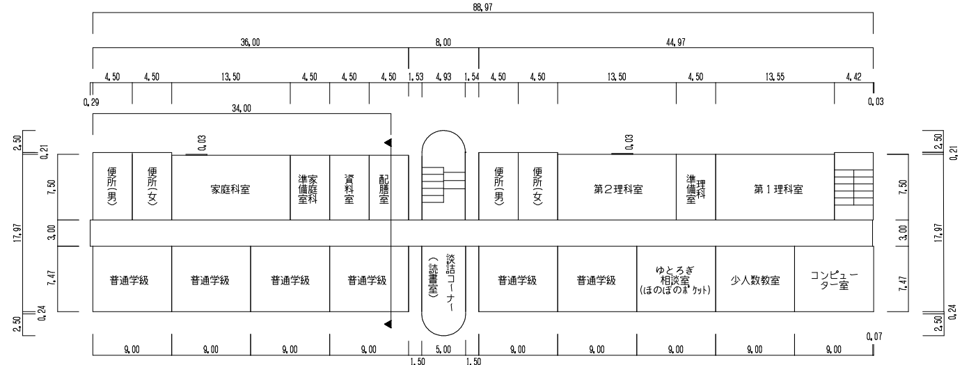
2階平面図
