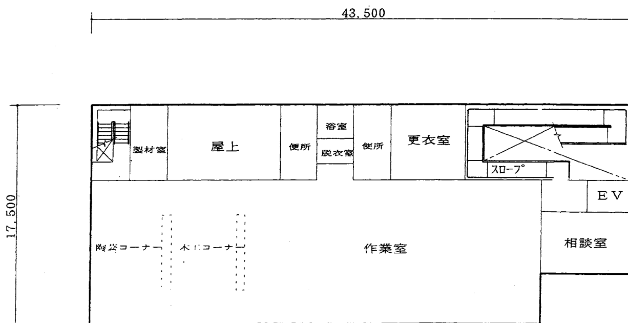
2階平面図
