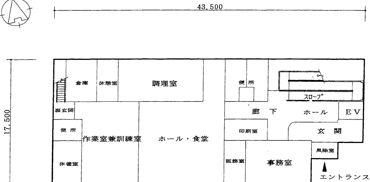
1階平面図
