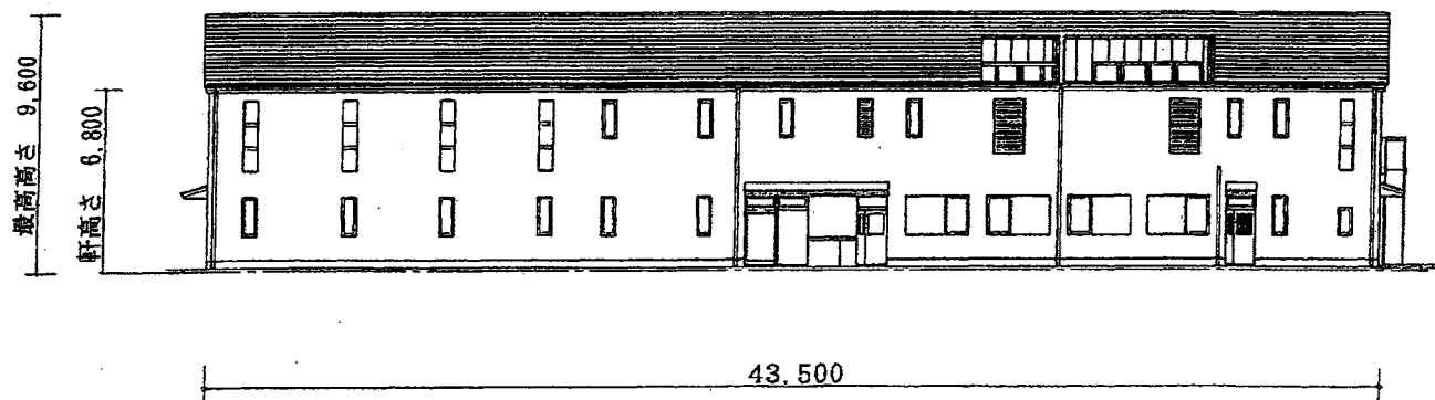
北立面図
