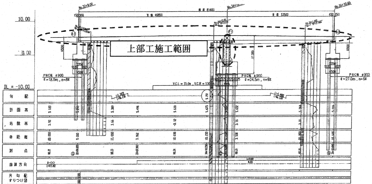
(仮)大柏川渡河部橋全体一般図
