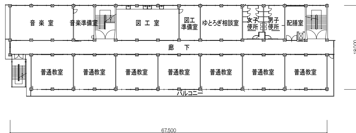
4階平面図
