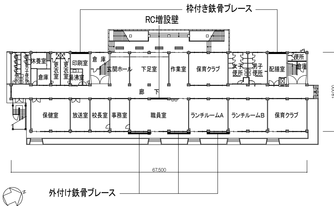
1階平面図
