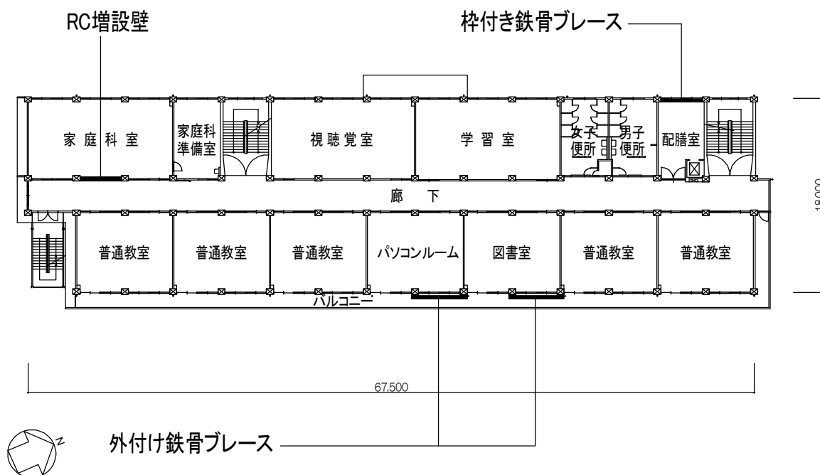
3階平面図
