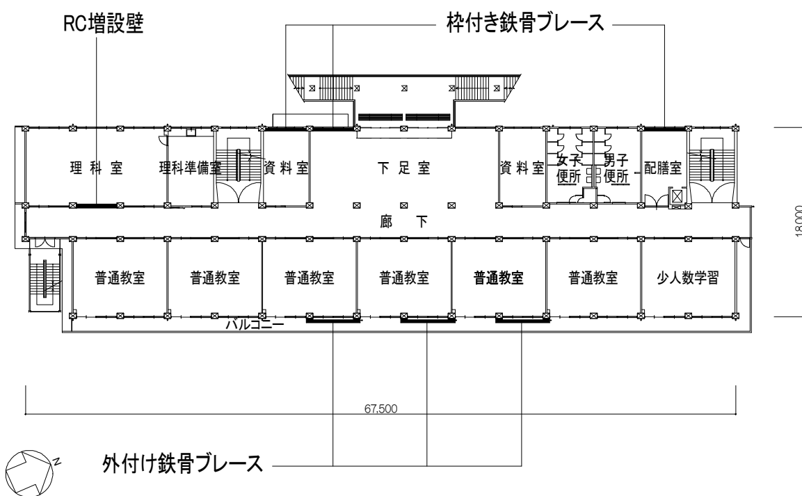
2階平面図
