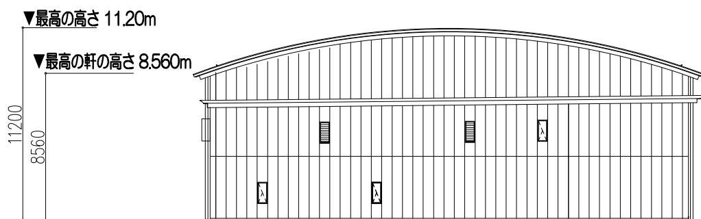
東側立面図
