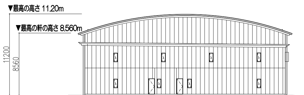
西側立面図
