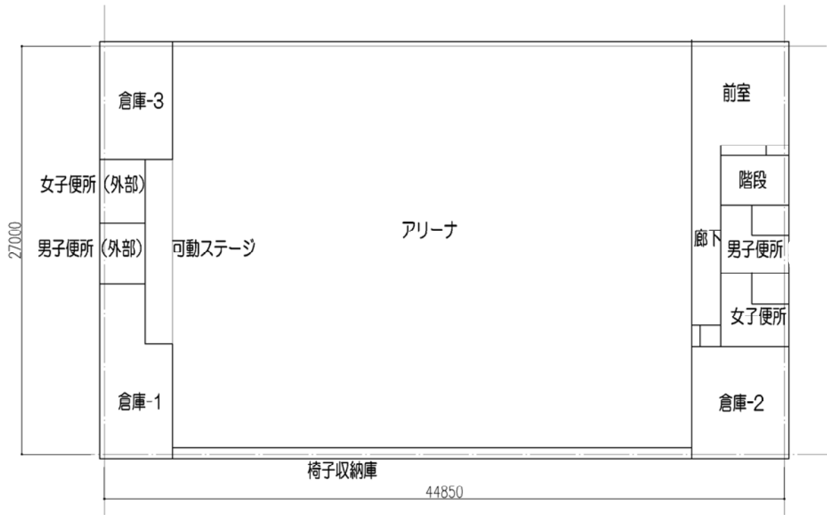
1 階 平 面 図
