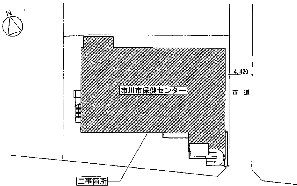
配置図
