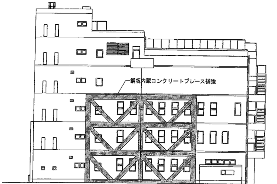
北側立面図
