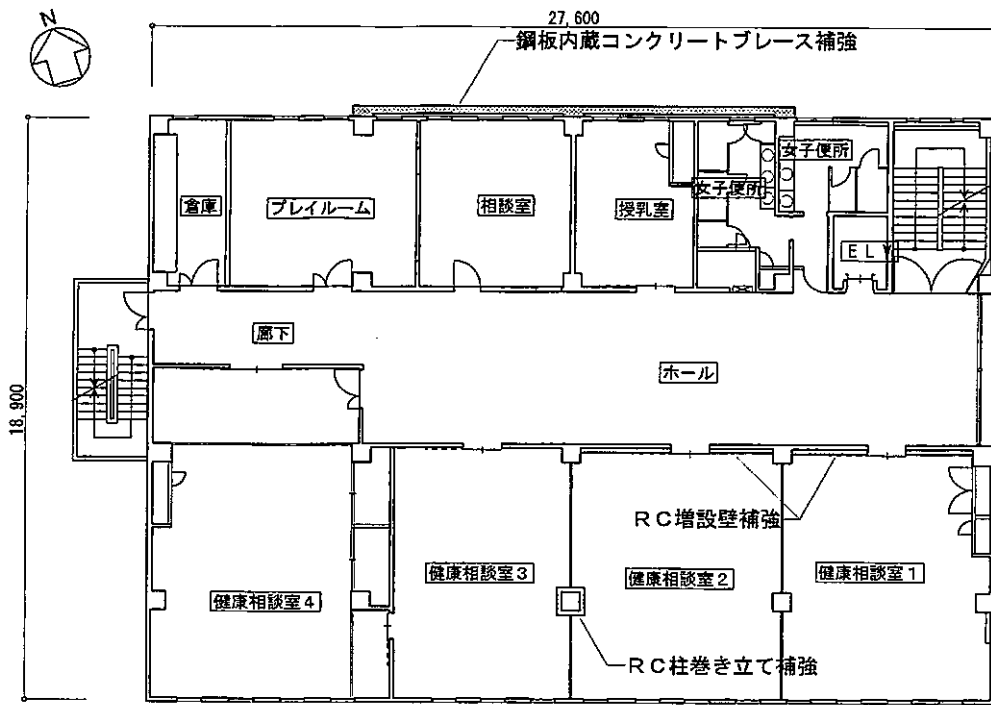
3階平面図
