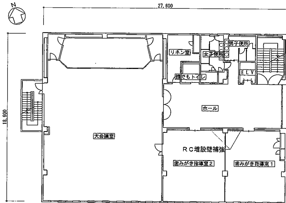
4階平面図
