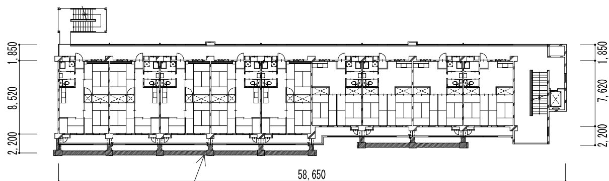
1 階平面図
