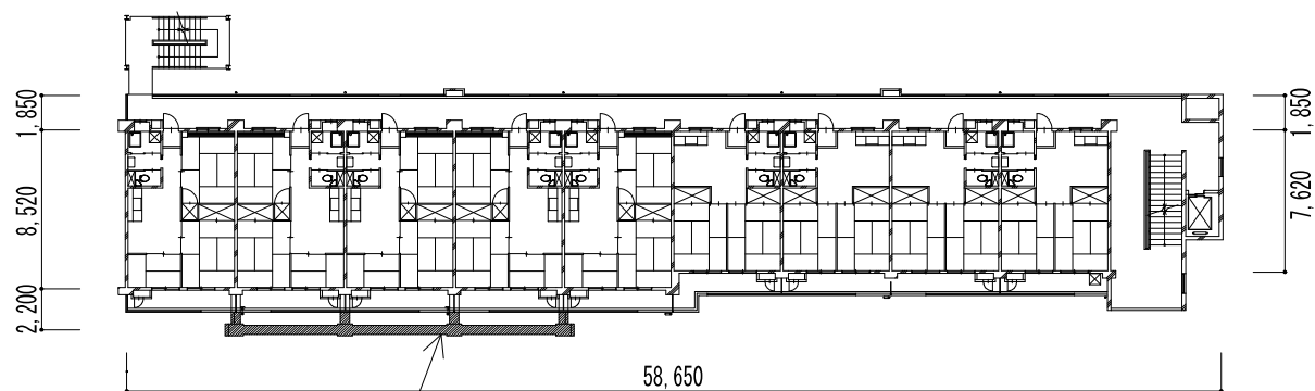
2 ～ 4 階平面図
