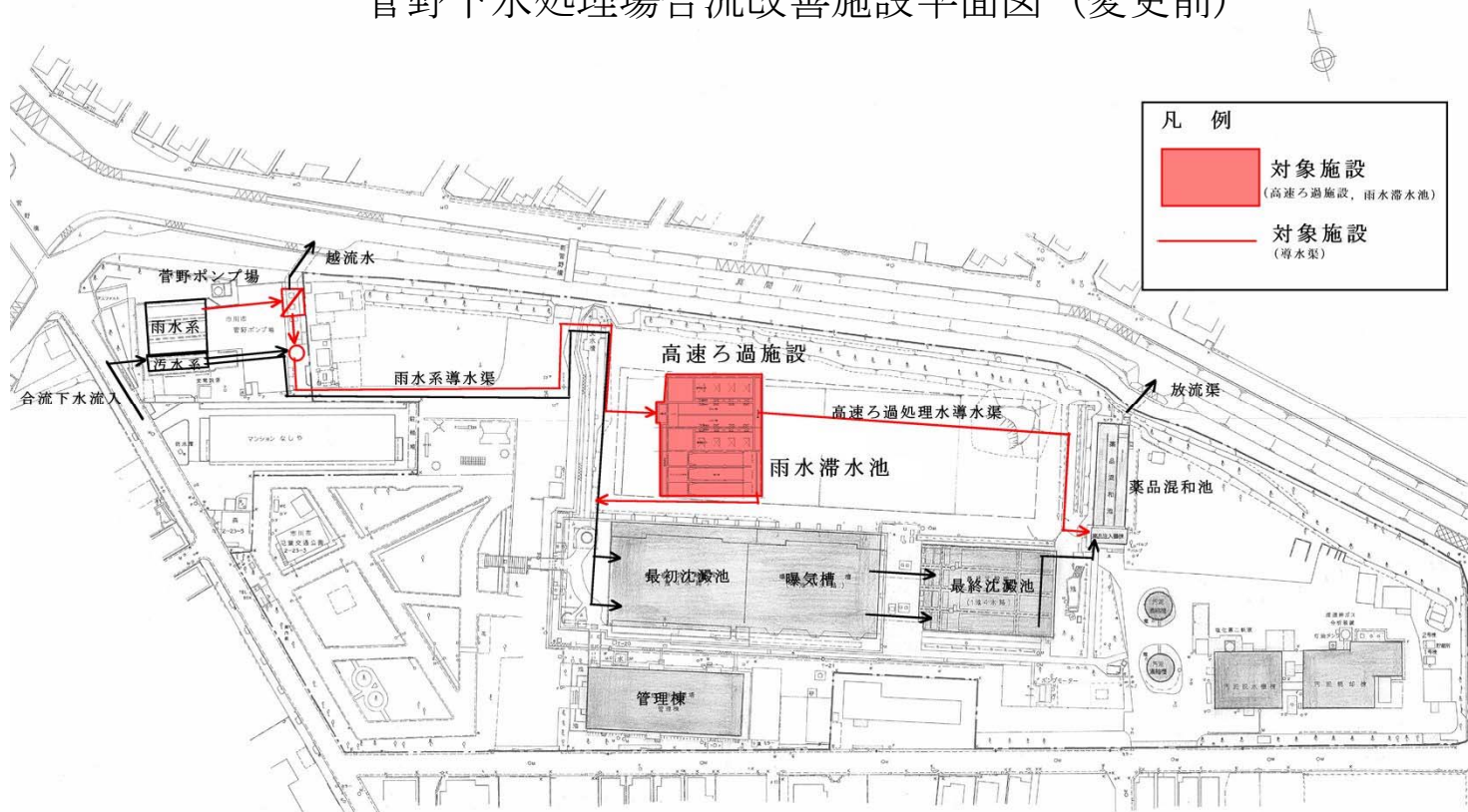
菅野下水処理場合流改善施設平面図（変更前）
