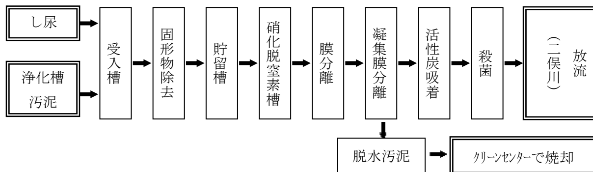
膜分離高負荷脱窒素処理フローシート
