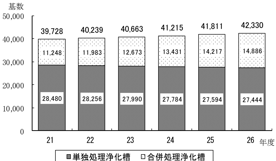
処理方式別浄化槽設置基数の推移
