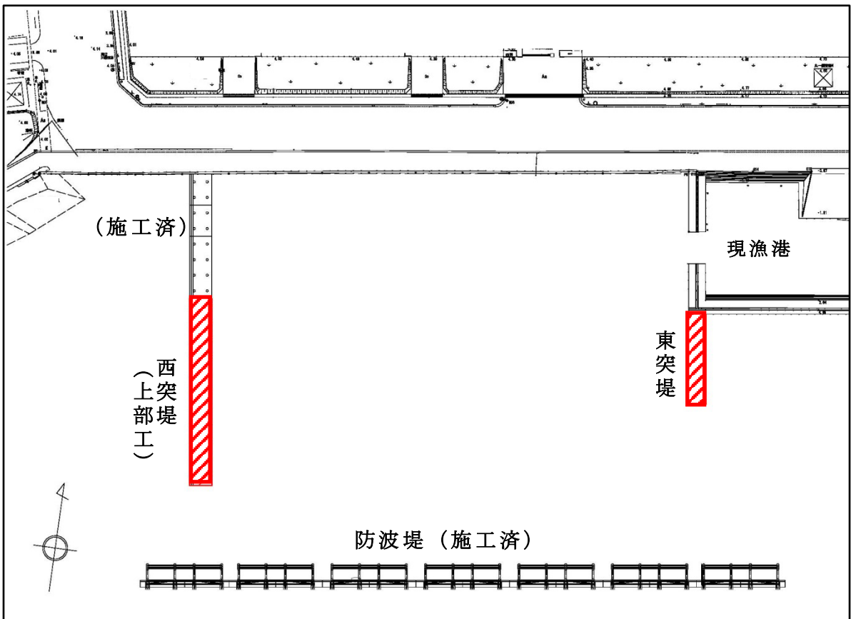
配置図
