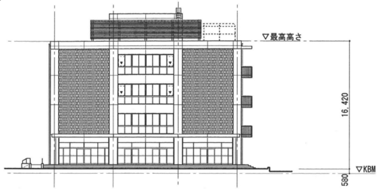
立面図（校舎棟 西面）
