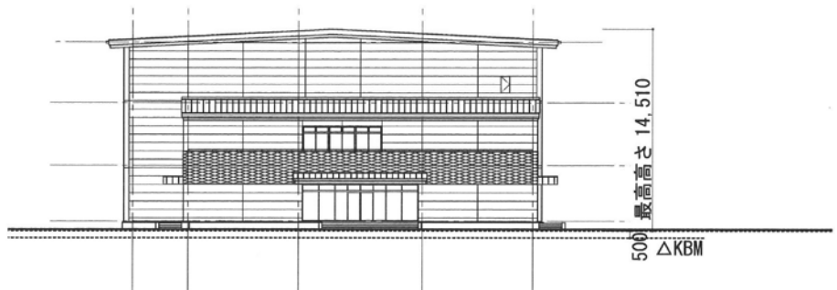
立面図（屋内運動場棟 西面）
