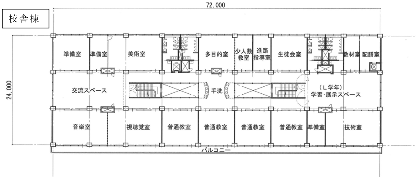
4階平面図
