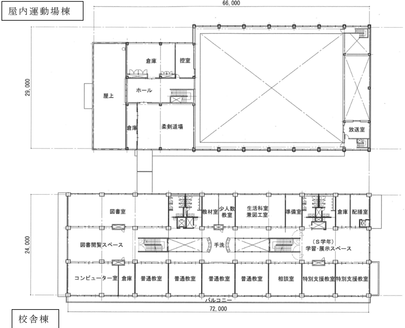
2階平面図
