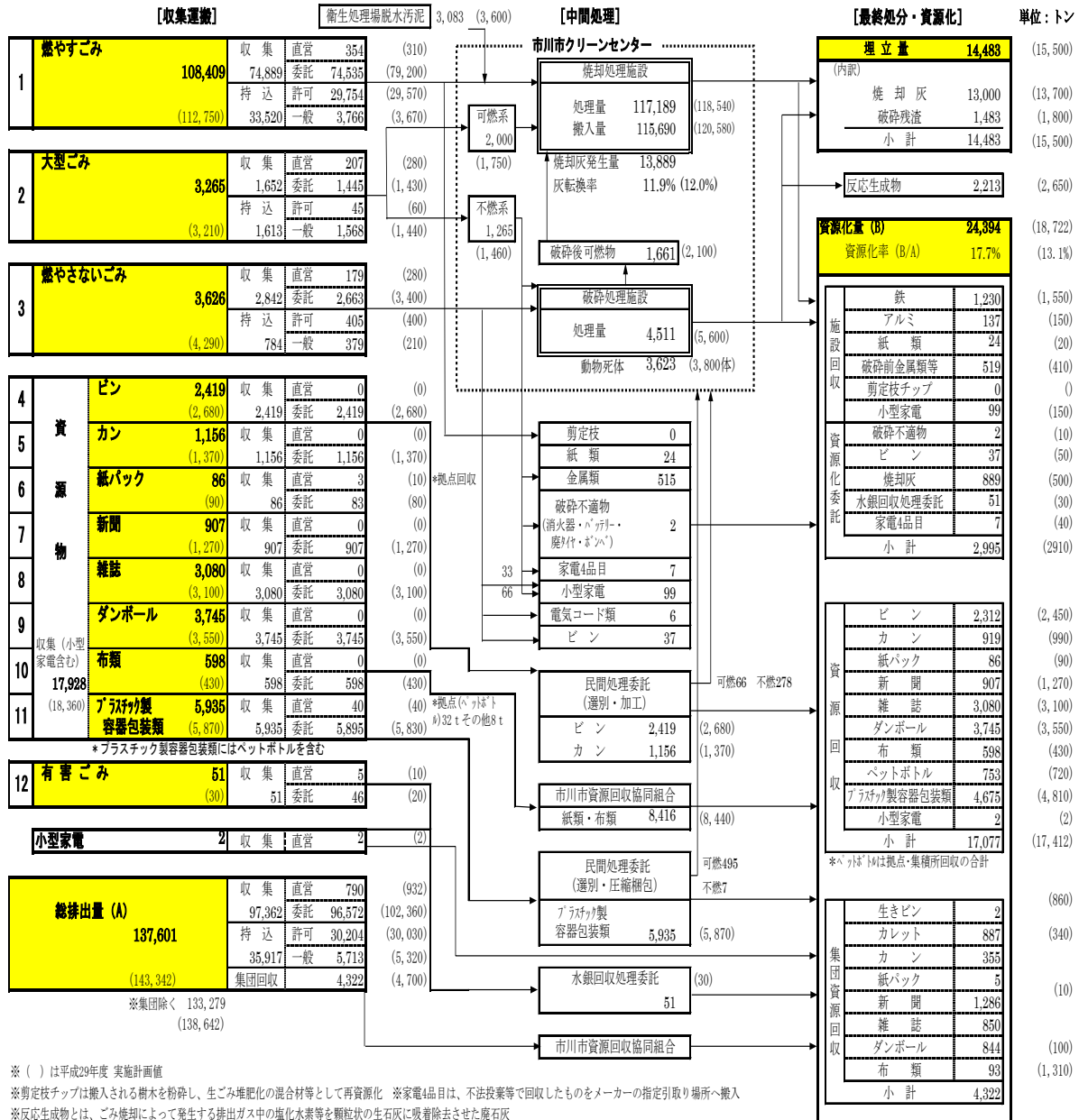
平成29年度 ごみ処理・資源物回収フローシート
