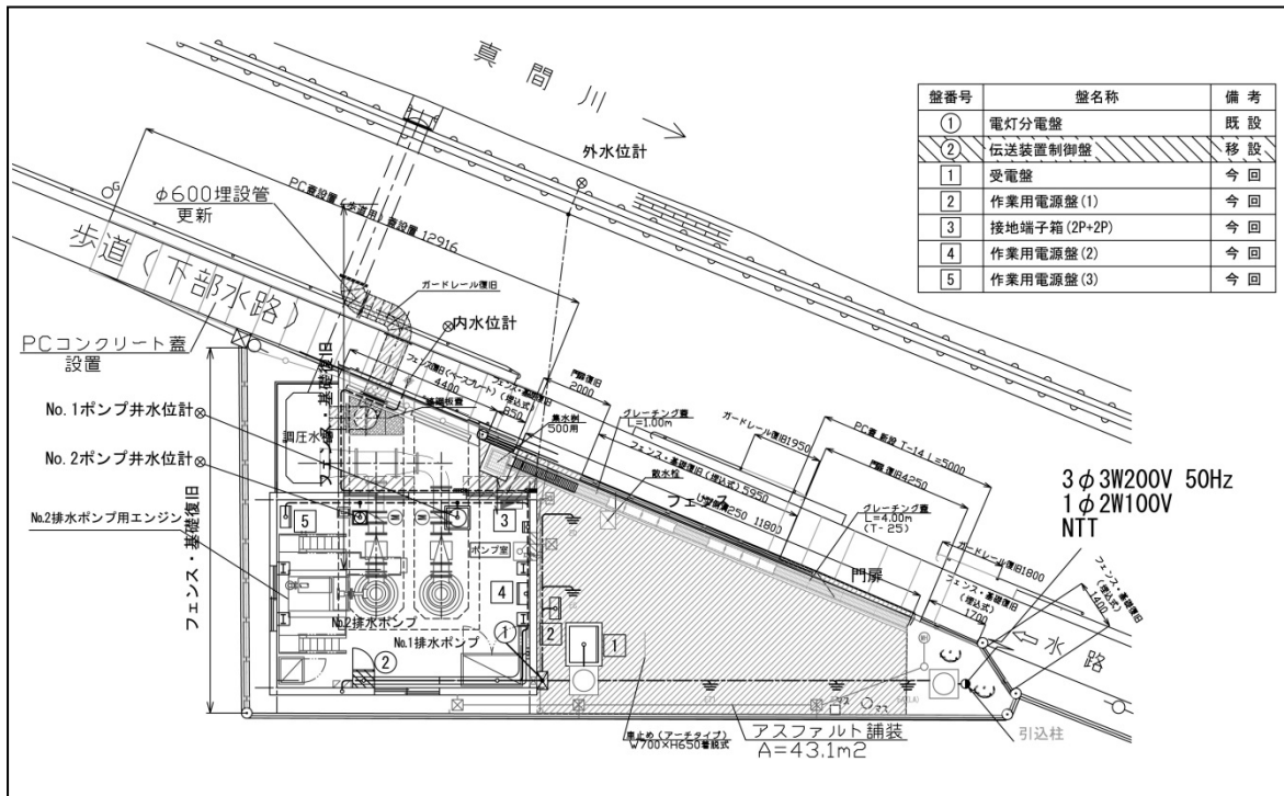
平面図
