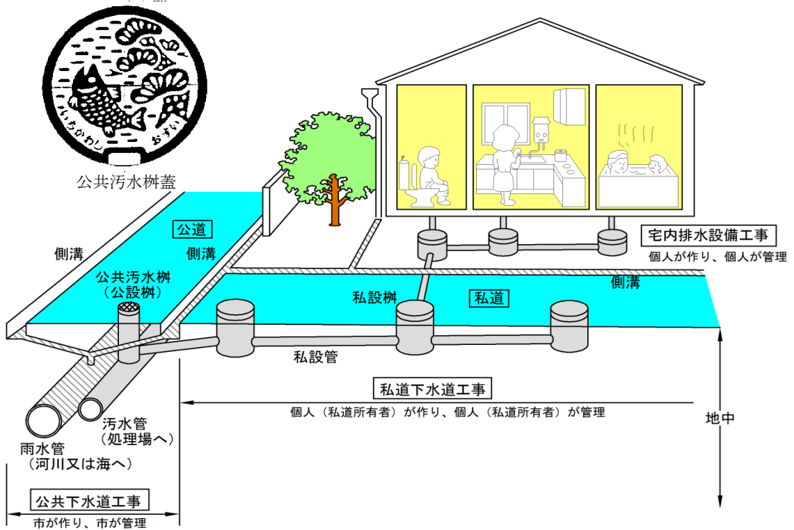
私道内の私設樹に接続する場合
