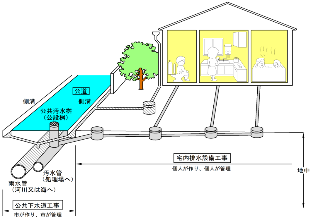
公道内の公設樹に接続する場合
