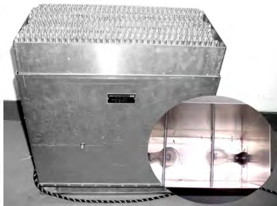
△2つのヒョコ電球(○内)が下から低温で熱し、乾燥させます。標本を挟んだ新聞紙とダンボール、アルミの波板を交互に挟んで空気の通りをよくしています。
