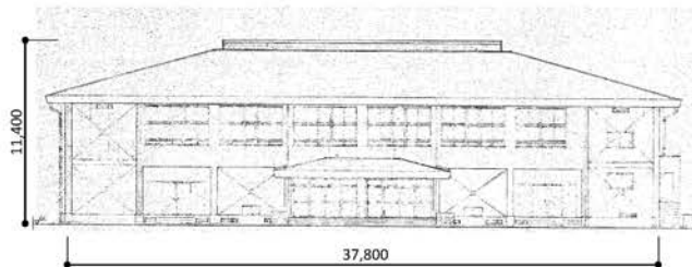
立面図（屋内運動場棟 北面）
