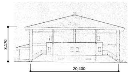
立面図（屋内運動場棟 西面）
