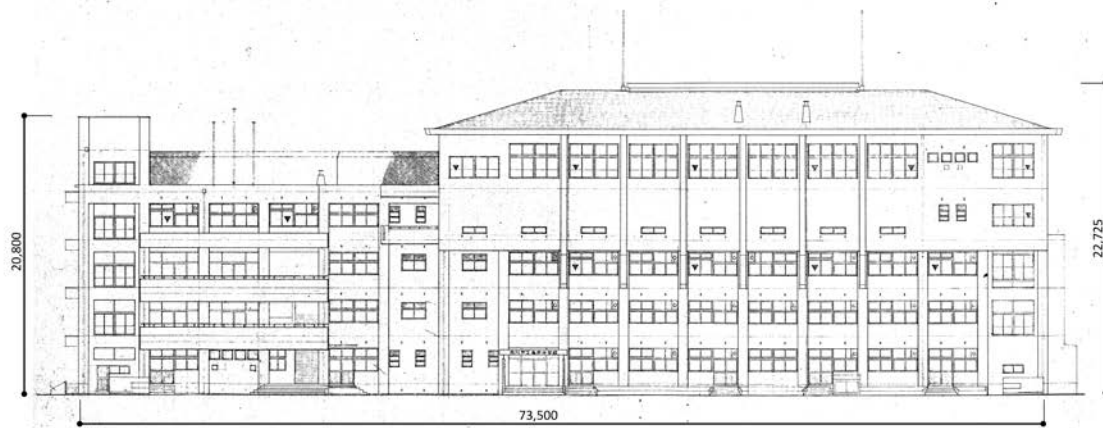
立面図（後期課程校舎棟 西面）
