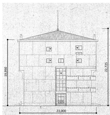
立面図（後期課程校舎棟 南面）
