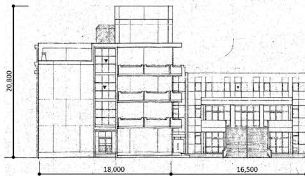
立面図（前期課程校舎棟・渡り廊下棟 南面）
