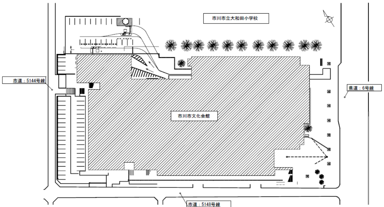
配置図
