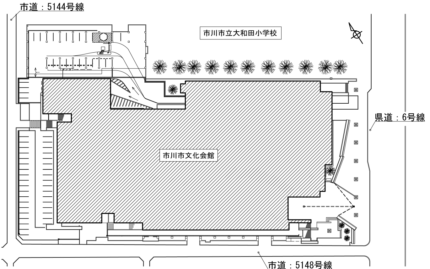
配置図
