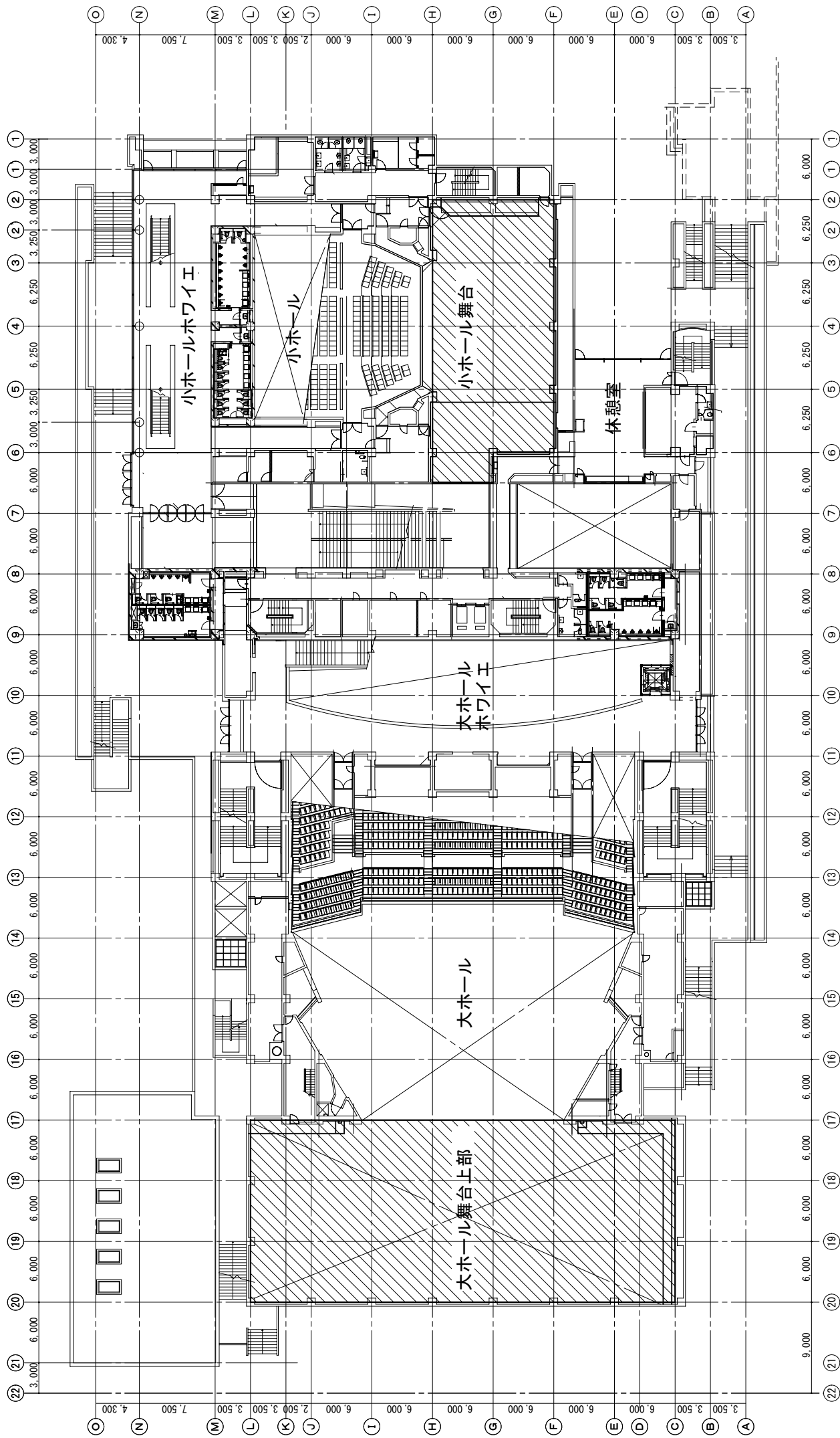
2階平面図
