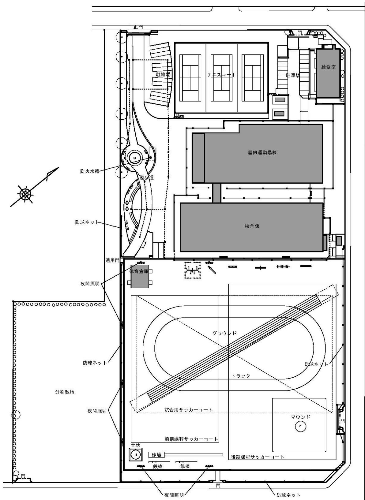
配置図
