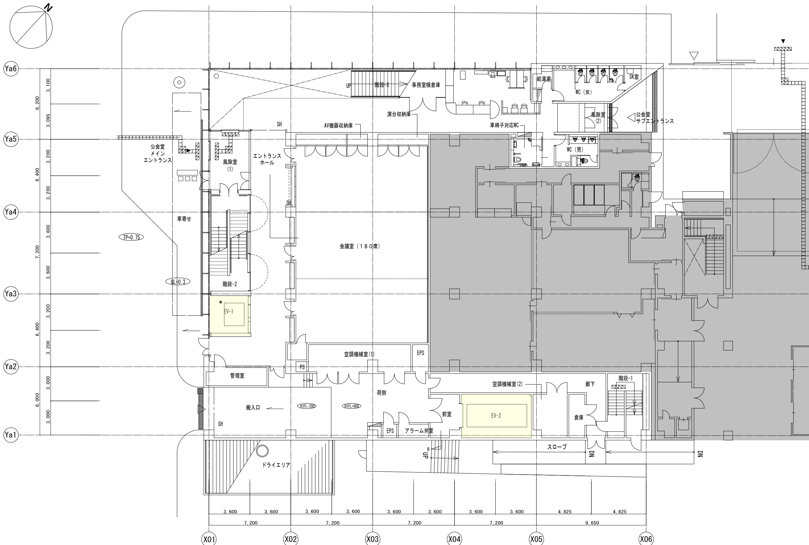
1階平面図
