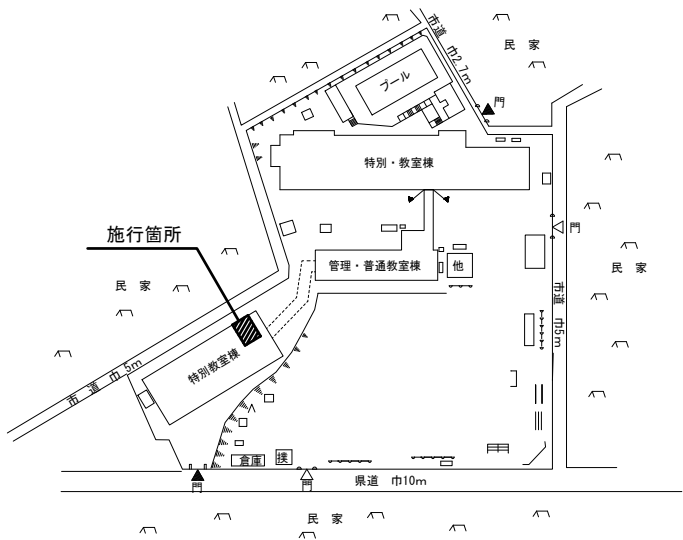
配置図 S=1/2500
