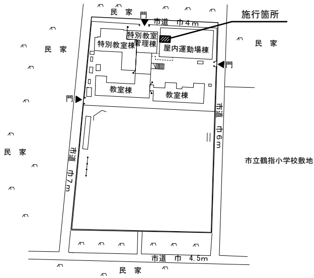
配置図 S=1/2500
