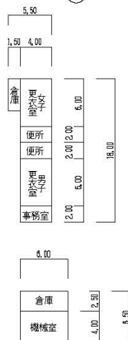
③③ プール付属室
