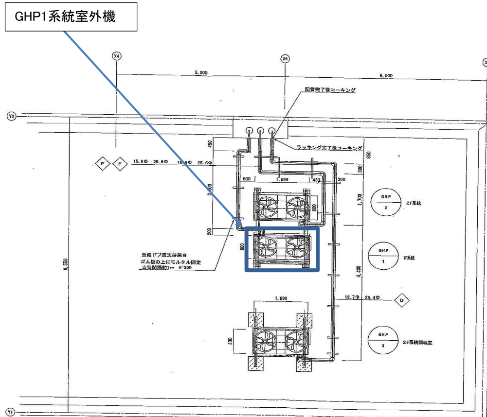
幸公民館屋上平面図
