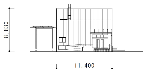
西側立面図
