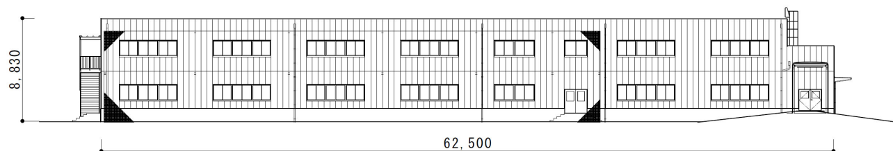
北側立面図
