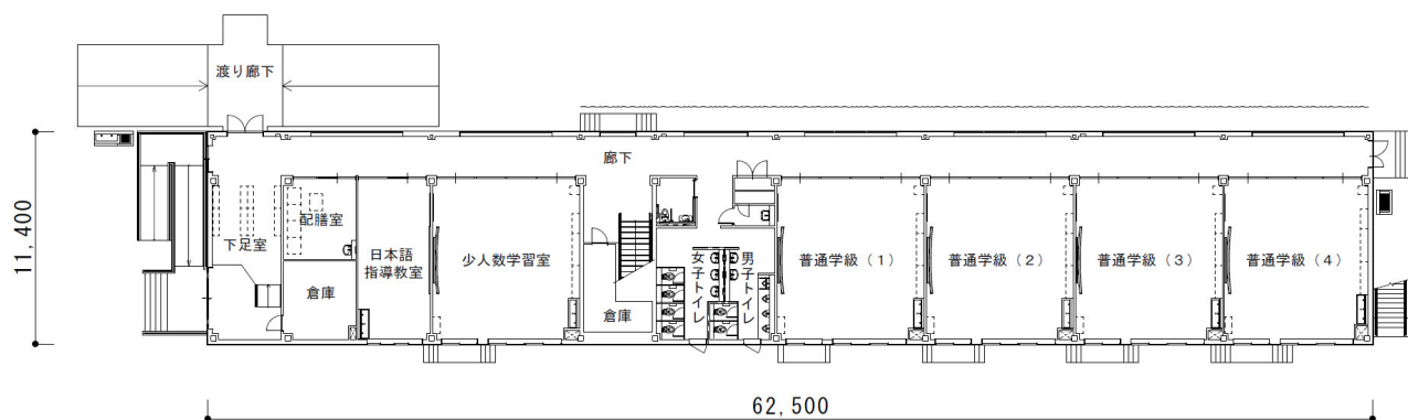
1階平面図
