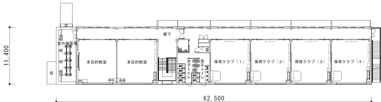
2階平面図
