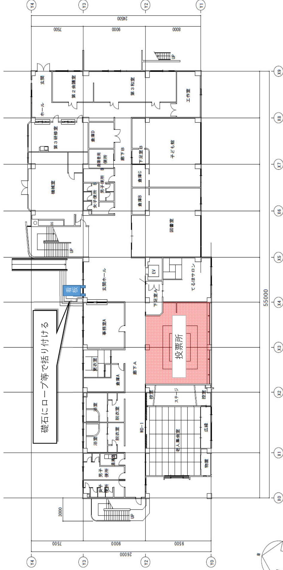
1階平面図
