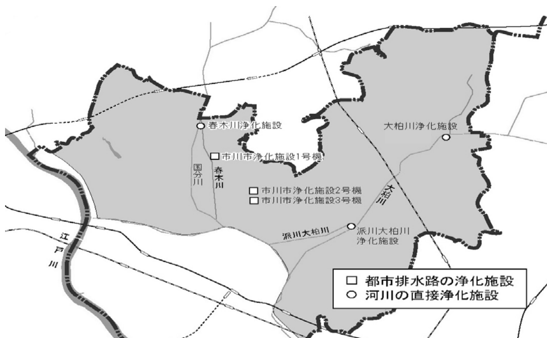
■ 浄化施設配置図
