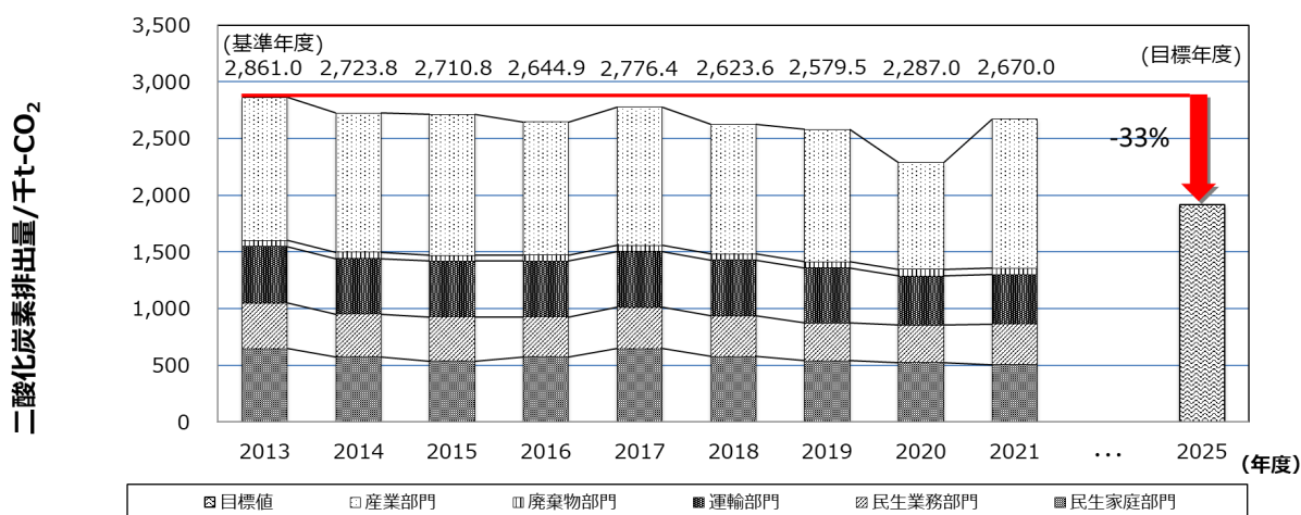
市川市の部門別二酸化炭素排出量の推移
