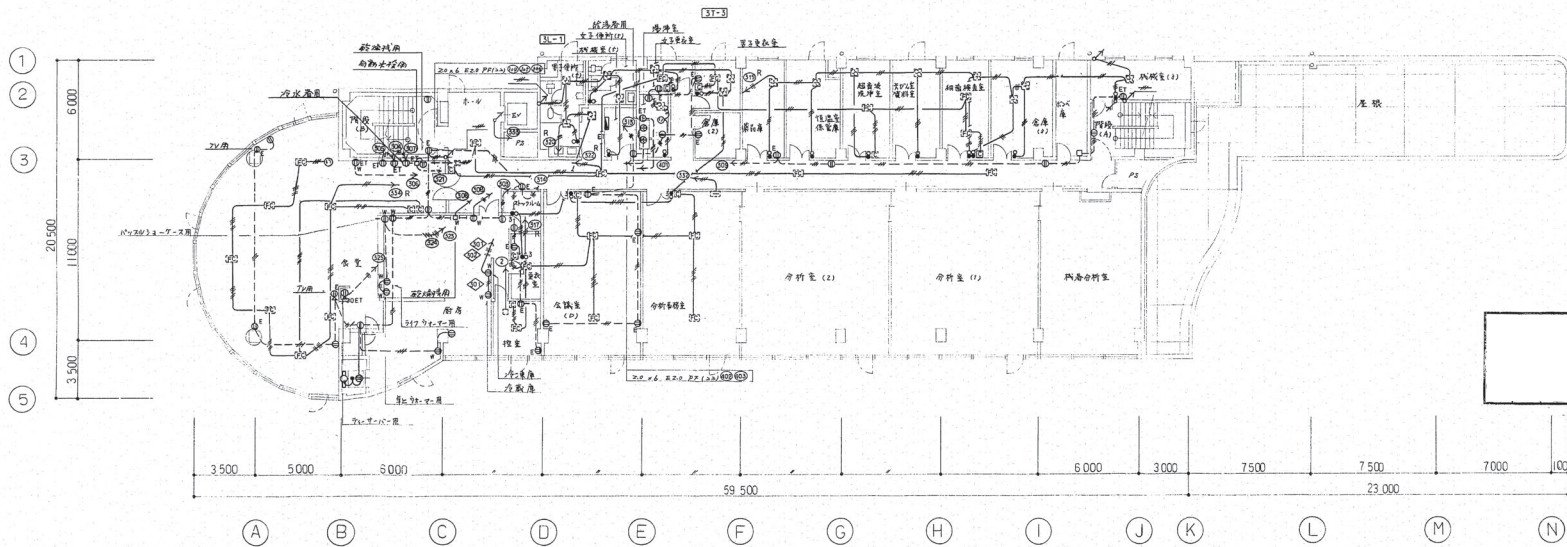
5楼平面图
