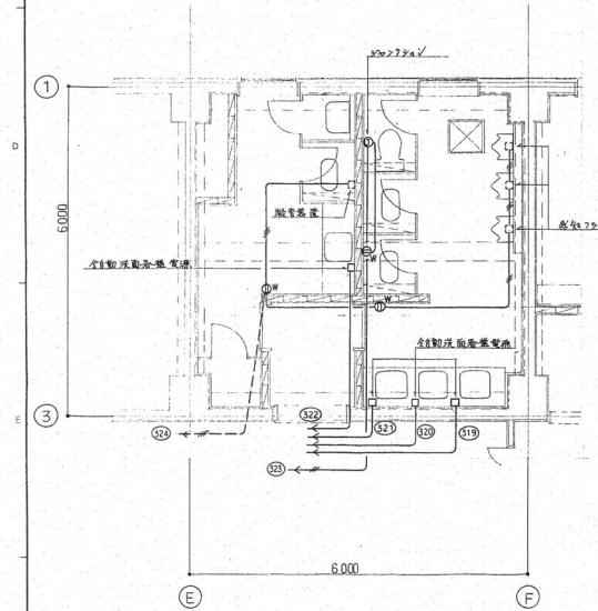
図略は 1L-1 ヱ 便所 (2) 平面詳細図
