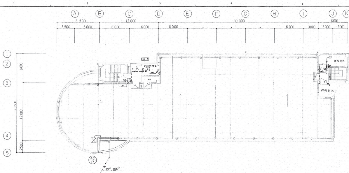
1楼平面图
