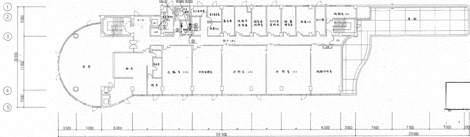
3階平面図
