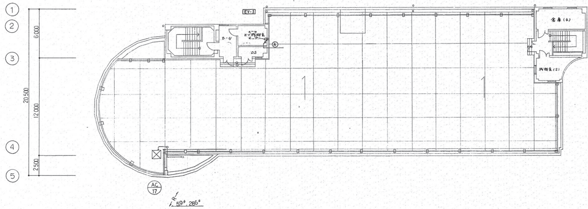
1階平面図
