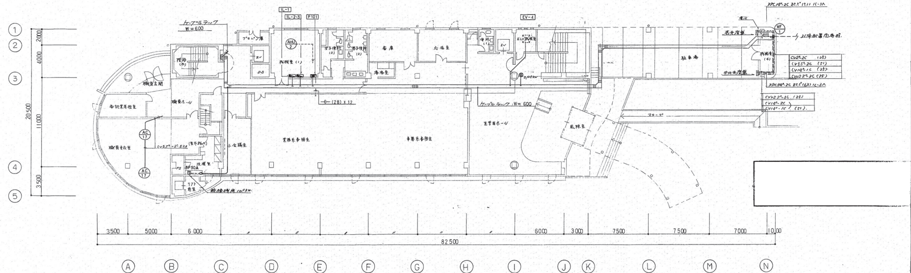
1階平面図
