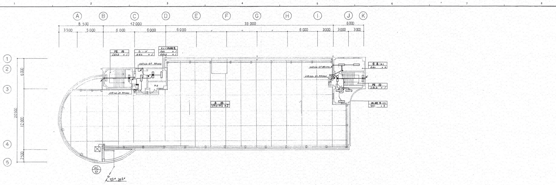
2楼平面图
