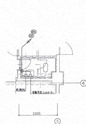
図略は 2L-1 ヱ 便所 (4) 平面詳細図
