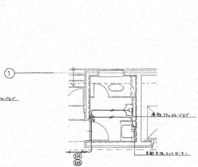
図略は 1L-1 ヱ 便所 (1) 平面詳細図
