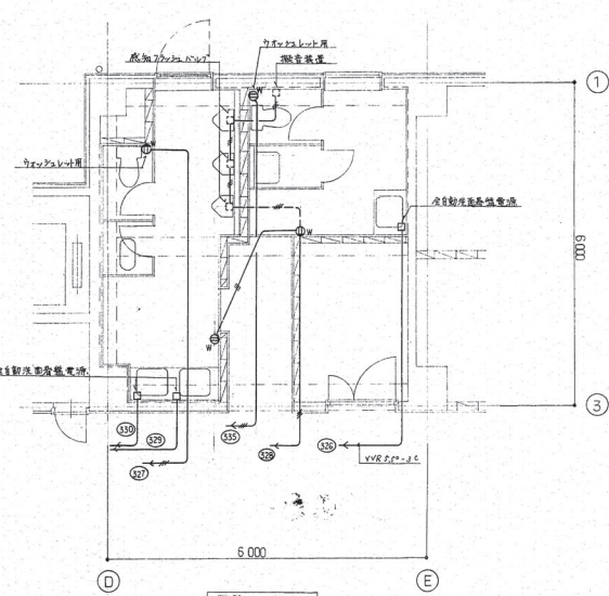
図略は 3L-1 ヱ 便所 (5) 平面詳細図
