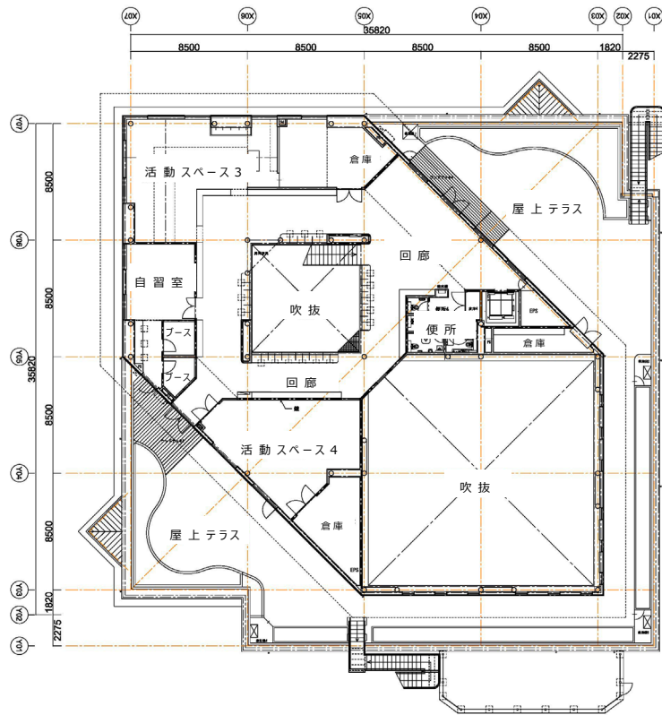
2階平面図
