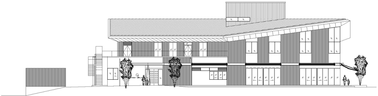
北西側立面図
