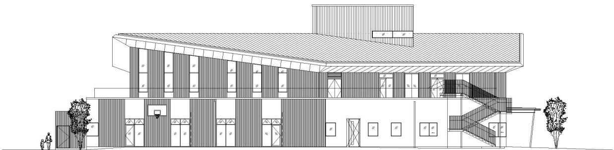
北東側立面図
