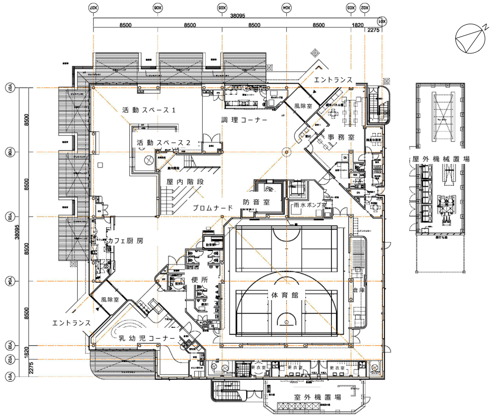
1階平面図
