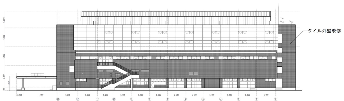
北側立面図
