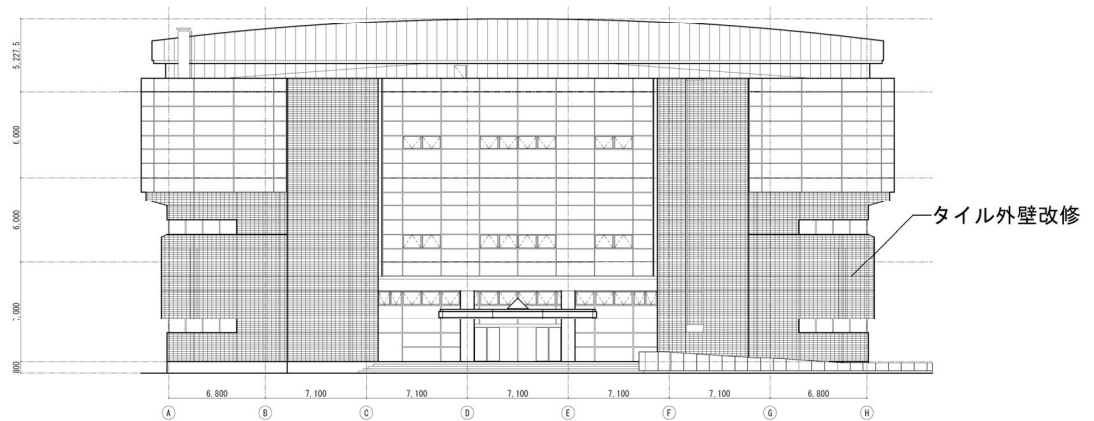
東側立面図
