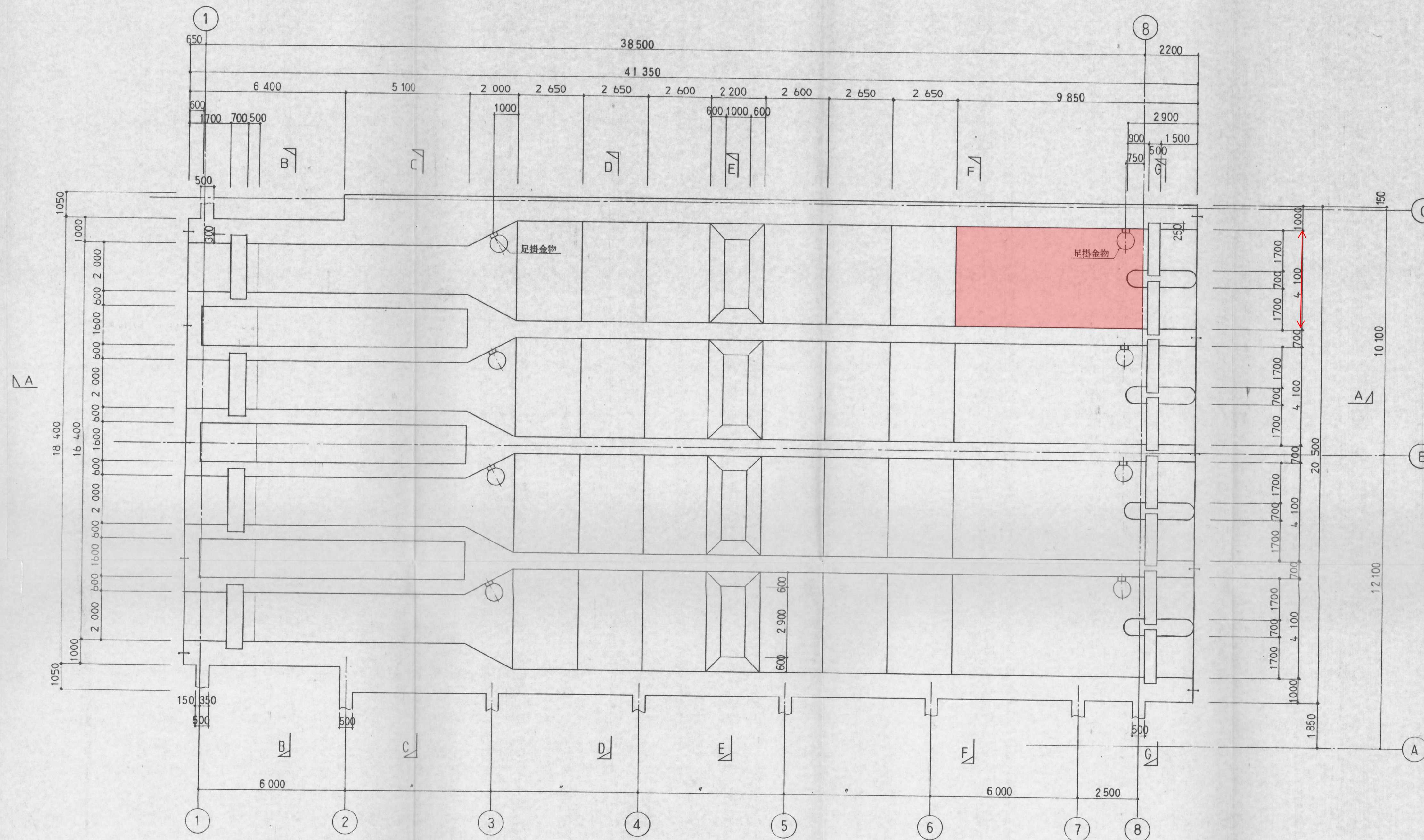
【浚渫箇所 沈砂池 平面図】
