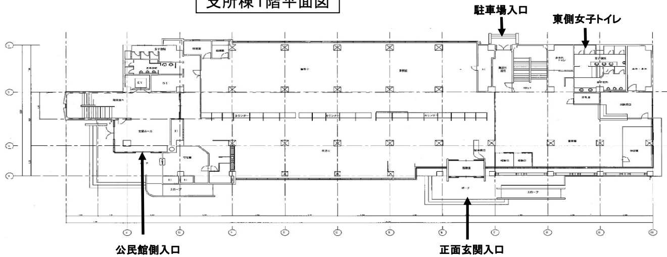
支所棟1階平面図
