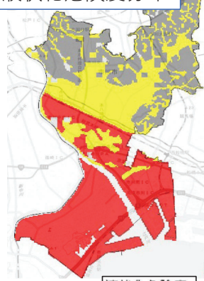
液状化危険度分布
