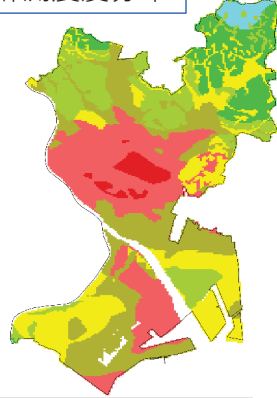
計測震度分布
