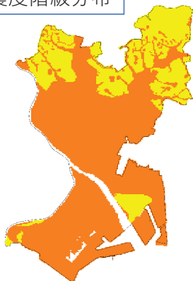
震度階級分布
