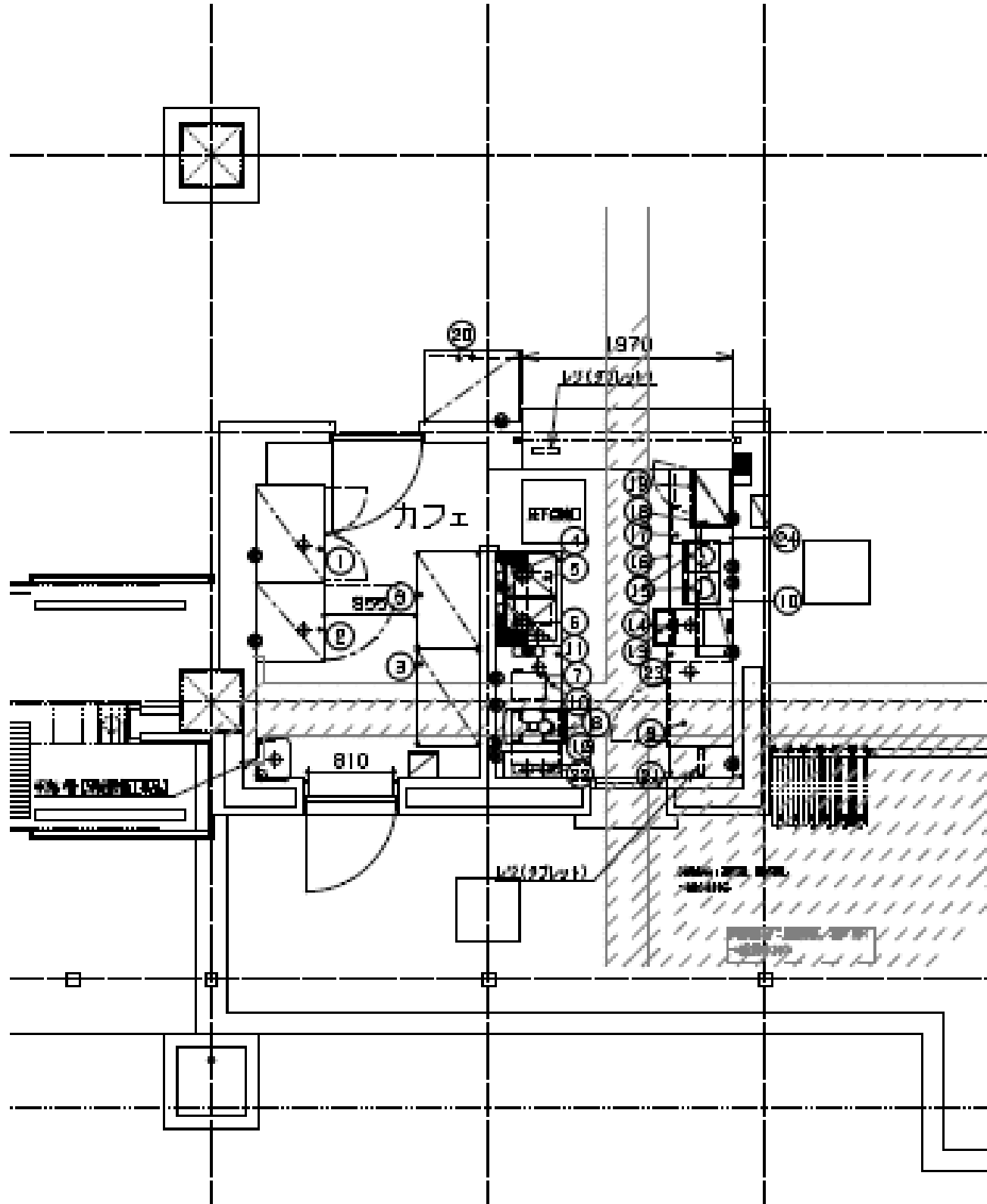
カフェスペース図面
