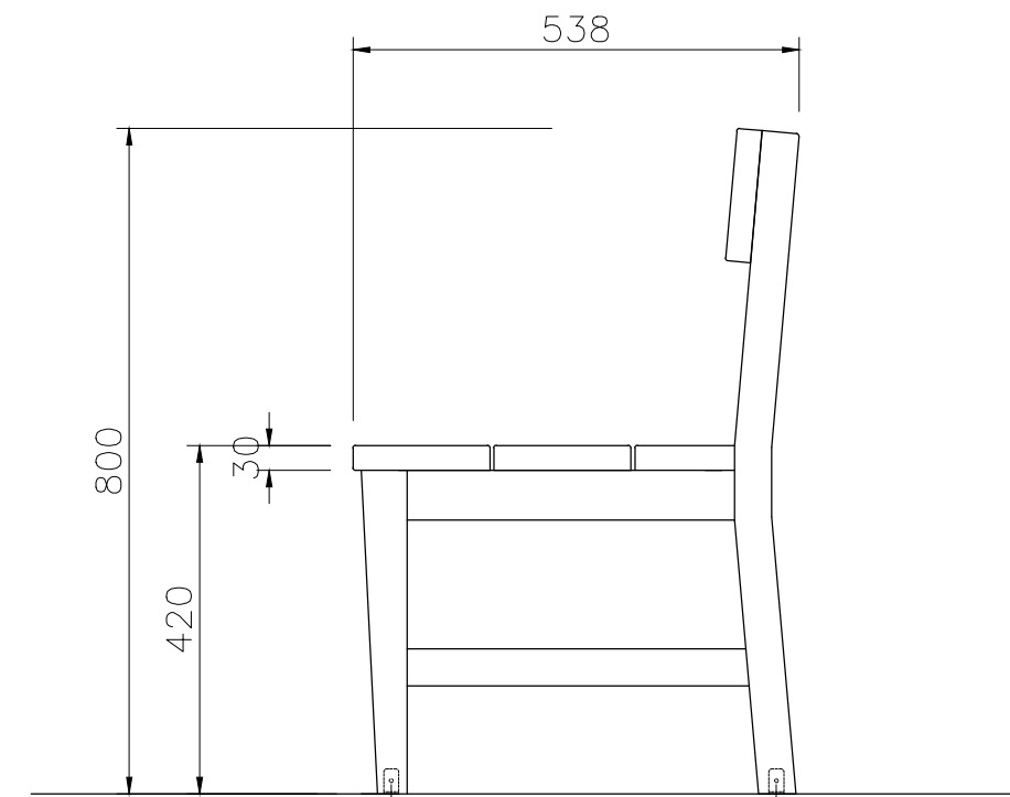
側面図
