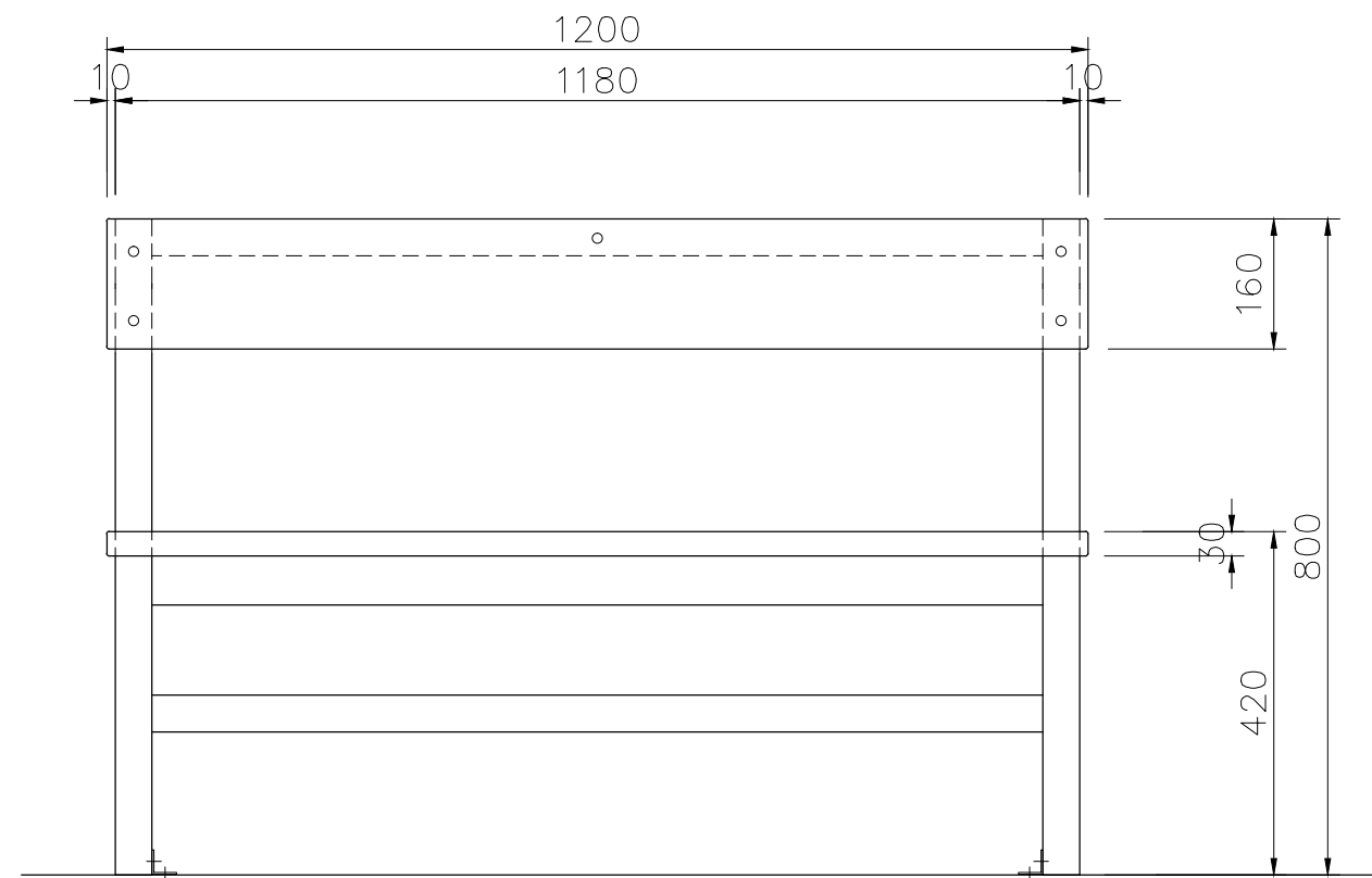
正面図
