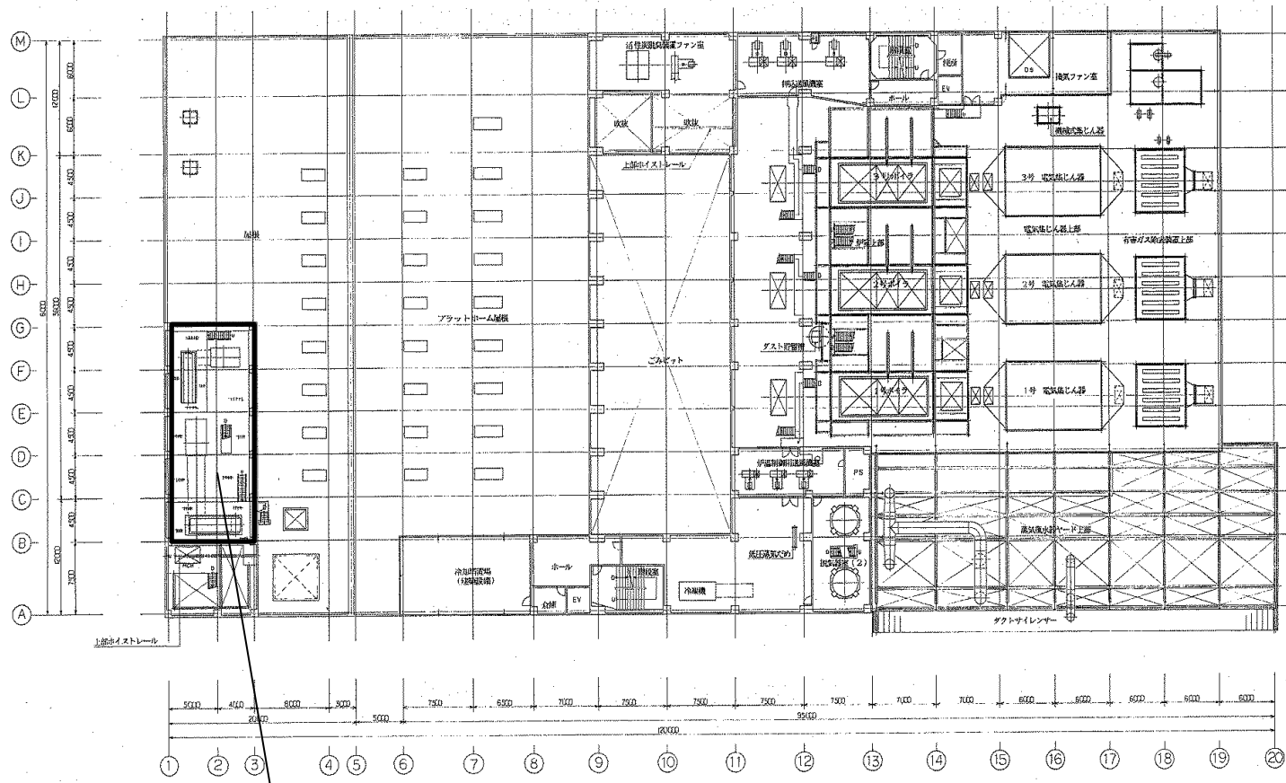
No.1可燃物搬送コンベアー室
